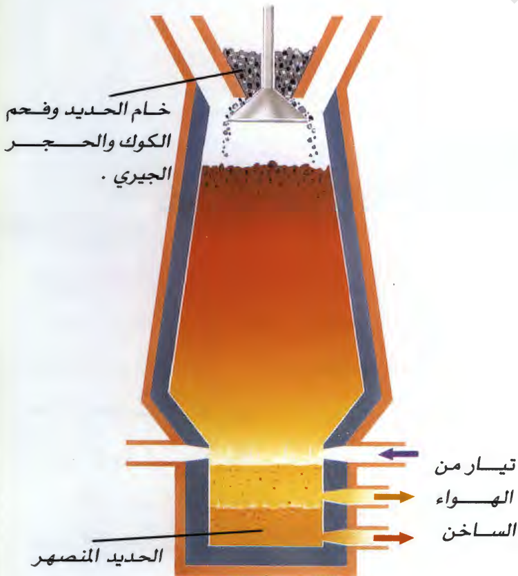
الفرن العالي
