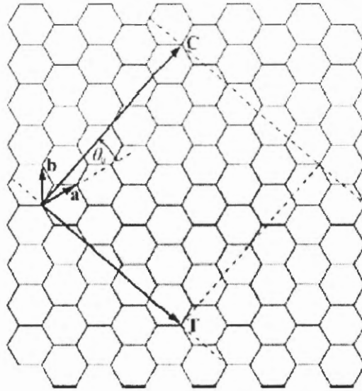
شكل (13) لوح جرافيت ذو بعدين يمكن ثنيه في اتجاه معين للحصول الأنبوب النانوي
