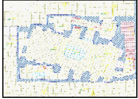
شكل ٣ - مسقط أفقي لرباط أزدرم - عن المجلس الأعلى للآثار
