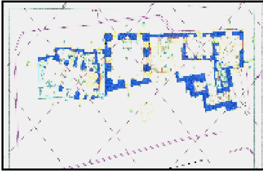
شكل ٢ - مسقط أفقى عام لمجموعة طراباى الشريفى ورباط أزدر إلى اليسار - عن المجلس الأعلى للآثار
