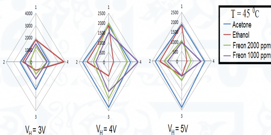
الشكل (10): بصمة الحساسات لأجل البارامتر t_s عند جهود تسخين مختلفة لأجل الأبخرة والغازات
