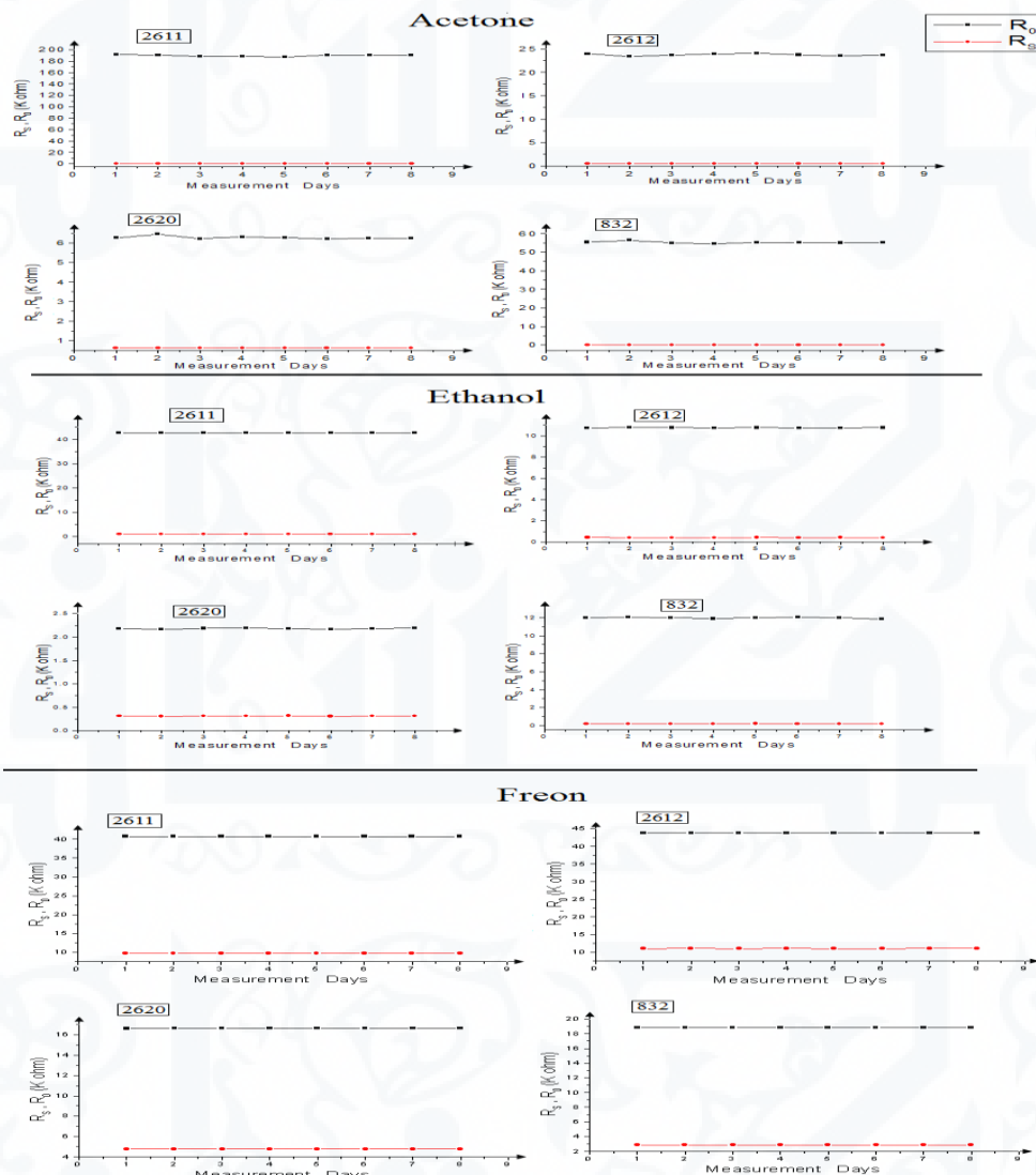
الشكل (4): حيد الحساسات متمثلاً بالبارامتر R_0
