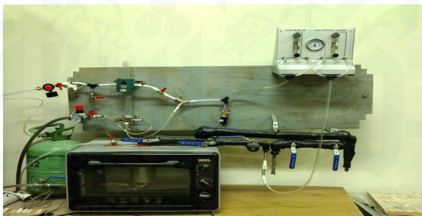
الشكل (2): الجهاز التجريبي المستخدم لتوصيف الحساسات لأجل الغازات
