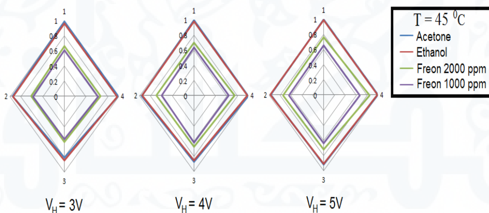
الشكل (8): بصمة الحساسات لأجل البارامتر S عند كمونات تسخين مختلفة لأجل الأبخرة والغازات
