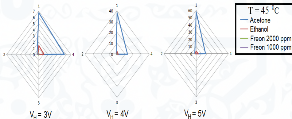
الشكل (9): بصمة الحساسات لأجل البارامتر Slope عند جهود تسخين مختلفة لأجل الأبخرة والغازات
