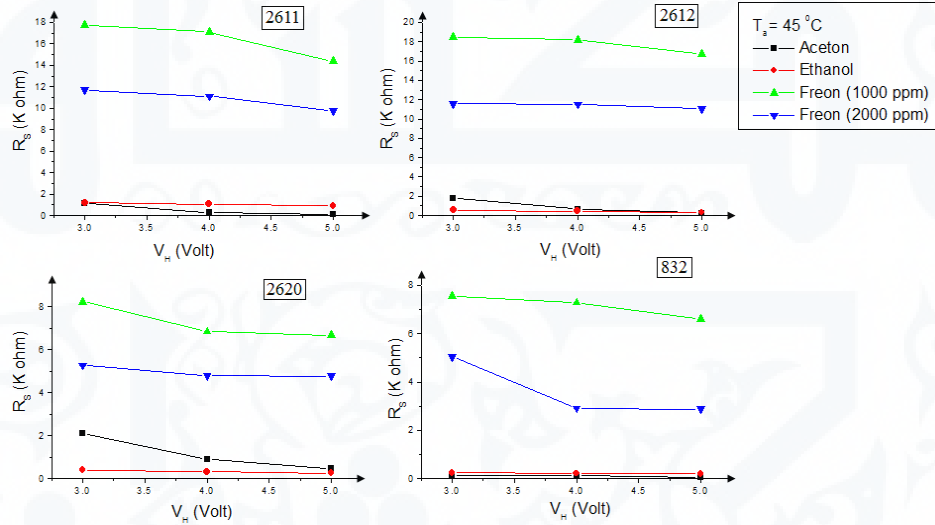
الشكل (5): تغير المقاومة المستقرة R_s مع زيادة جهد تسخين V_H للحساسات وعند درجة حرارة T_a = 45^\circ\text{C} للوسط المحيط بالحساسات لأجل الأبخرة والغازات معاً
