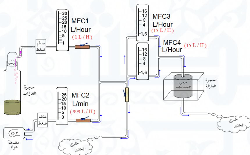
الشكل (3): المخطط التفصيلي للجهاز المستخدم للكشف عن غاز الفريون
