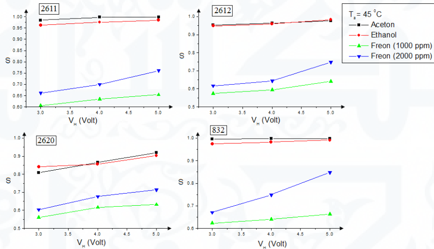
الشكل (6): تغير التحسسية S مع زيادة جهد تسخين V_H للحساسات وعند درجة حرارة T_a = 45^\circ\text{C} للوسط المحيط بالحساسات لأجل الأبخرة والغازات معاً
