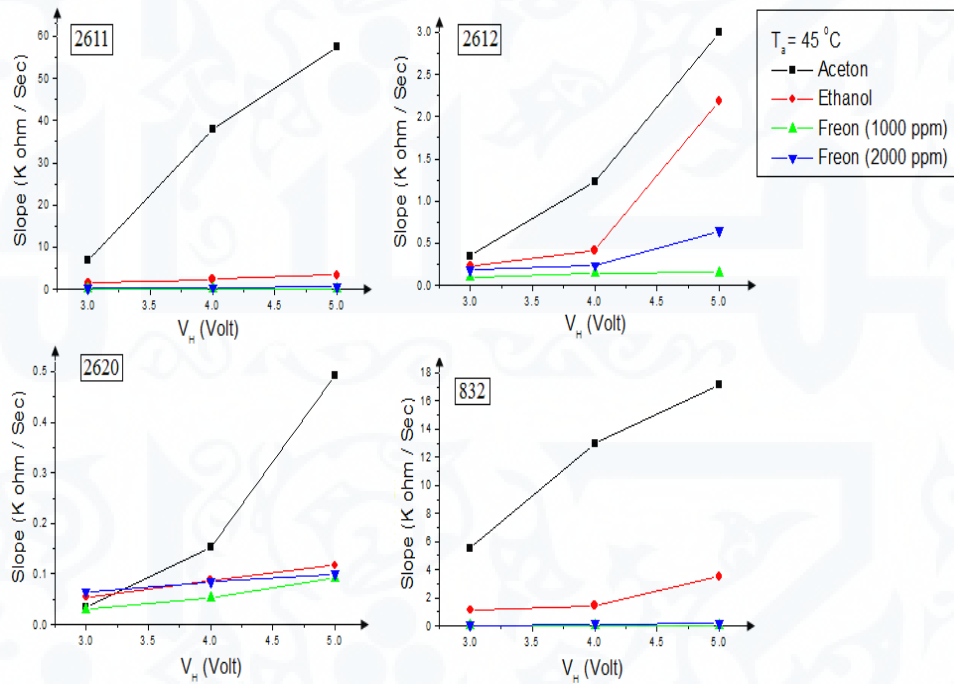
الشكل (7): تغير سرعة الإستجابة التحسسية Slope مع زيادة جهد تسخين V_H للحساسات وعند درجة حرارة T_a = 45^\circ C للوسط المحيط بالحساسات لأجل الأبخرة والغازات معاً
