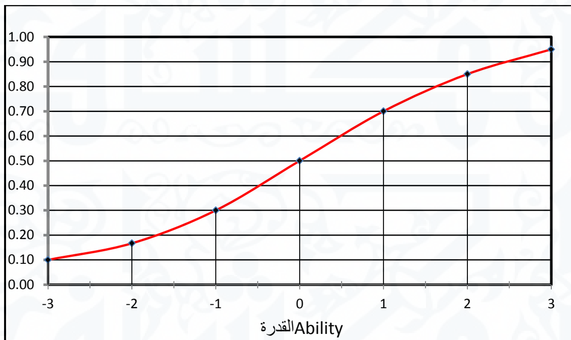
الشكل (3) المنحنى المميز للاختبار (الصيغة النهائية)
