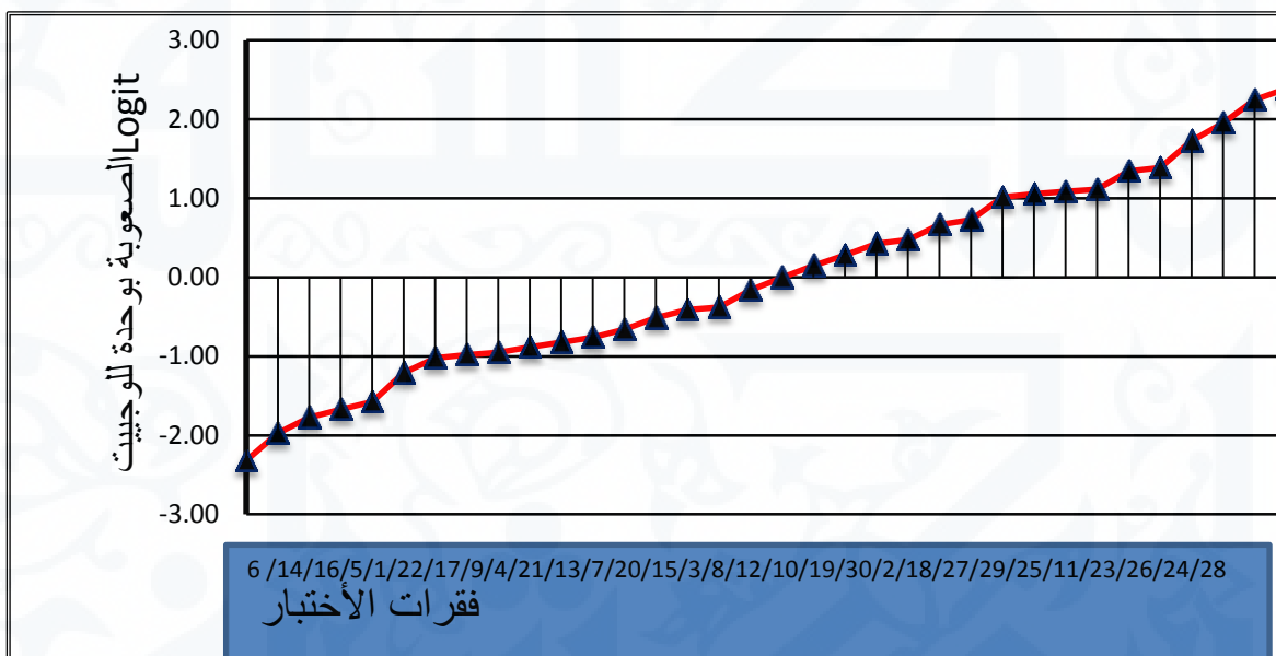
الشكل (1) تدرج فقرات الاختبار (الصيغة النهائية) وبحسب تقديرات الصعوبة بوحدة اللوجيت .Logit
