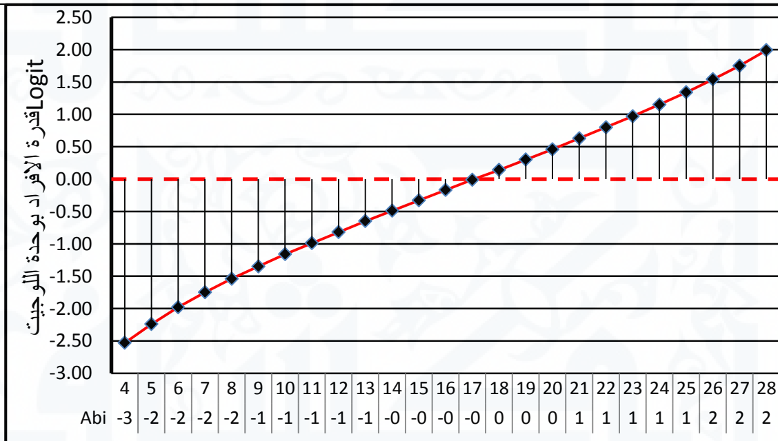
الشكل (2) تدرج قدرات أفراد العينة والمقدرة بوحدة اللوجيت .Logit
