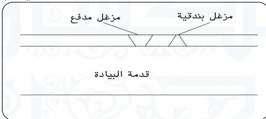
شكل (١٦) مسقط أفقي تحليلي لجزء من احدى أسوار الخانقاه النظامية موضح عليه قدم بيادة ومزل بندقية ومزل مدفع (رسم بمعرفة الباحث)
