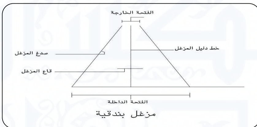
شكل (١٧) مسقط أفقي تحليلي لمزل البندقية (رسم بمعرفة الباحث)
