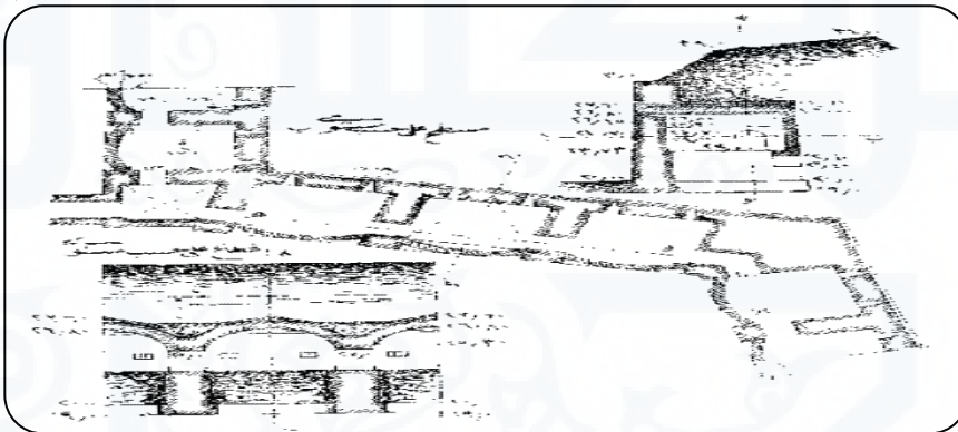
شكل (١٩) مسقط أفقي وقطاع رأسي لجزء من سور موضح عليه مزاغل البنادق (عن مخطوط المطالع القمرية في الأبنية العسكرية - مكتبة المتحف الحربي)
