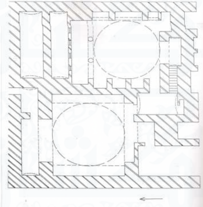
مخطط (١) مخطط ارضي لحمام سعيد الشروفي
