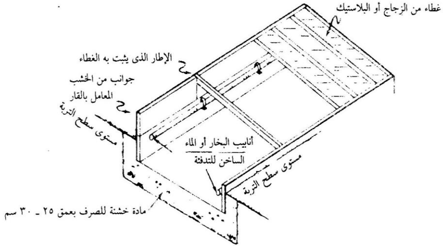
شكل (١٣-٣): المراقد المدفأة Hotbeds (عن Boodley ١٩٨١).
