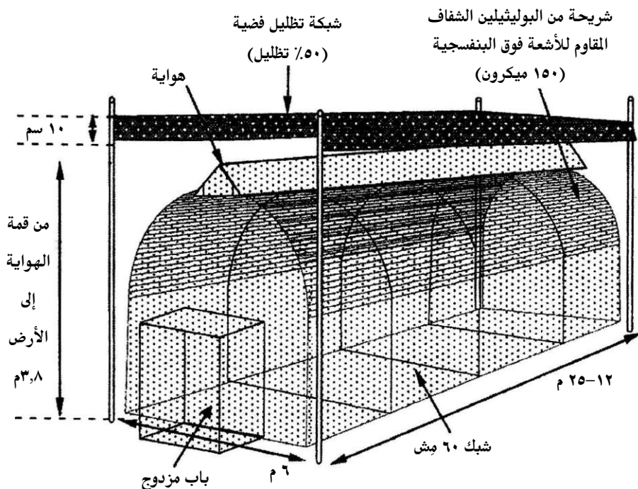
شكل (٩-١): تخطيط لصوبة سلكية تناسب إنتاج الشتلات المطعومة.
