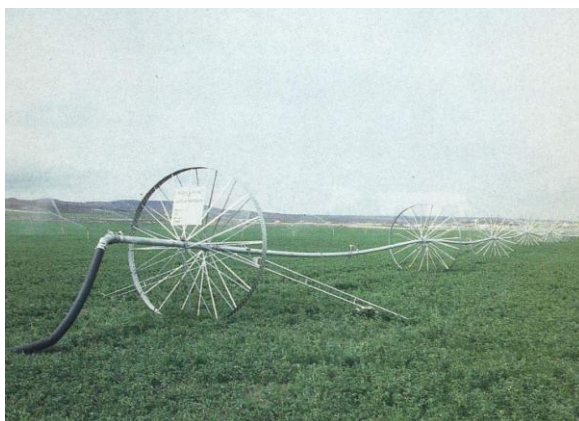
شكل (١١-١٦): الري بالرش بنظام الأنابيب المتحركة على عجل.
