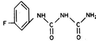
Fluorophenylbiuret
