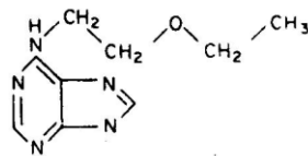
Ethoxvethyladenine
