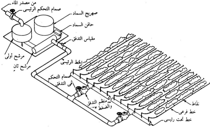
شكل (١٦-١٤): شبكة الري بالتنقيط.
