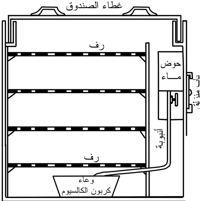
شكل (20): رسم تفصيلي لصندوق التلوين بغاز الأسثيلين.
