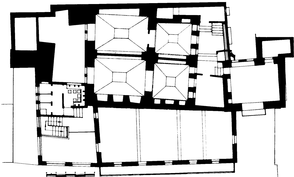
قسم الآثار الإسلامية - القدس مسجد أبي يحيى الصديق - خربة جنة - بيت الخزينة - مقياس ١:٨٠٠ تم إنشاؤه في القرن الرابع الهجري بقايا الخندق - حنّ أبو قلدش
