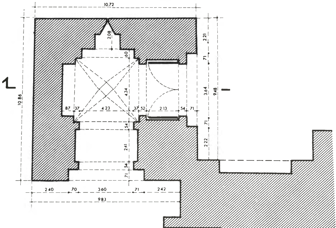
مسطح أفقي
