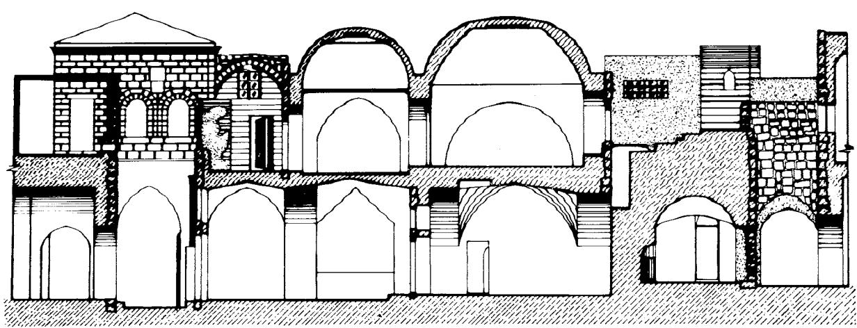
قسم الآثار الإسلامية - القدس مسجد أبي يحيى الصديق - بيت الخزينة المقياس ١:٨٠٠ تم إنشاؤه في القرن الرابع الهجري بقايا الخندق - حنّ أبو قلدش
