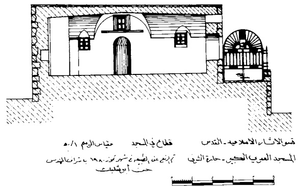
قطاع طولي
