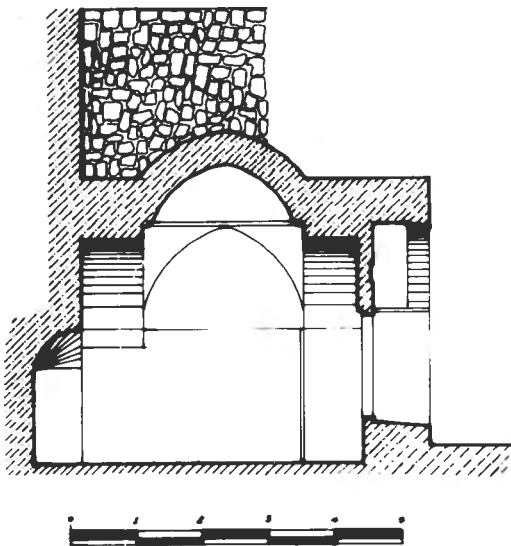
قسم الآثار الإسلامية - القدس مسجد الشورى - القدس قطاع ١.١ تم إرفاقه مع الخريطة تان
