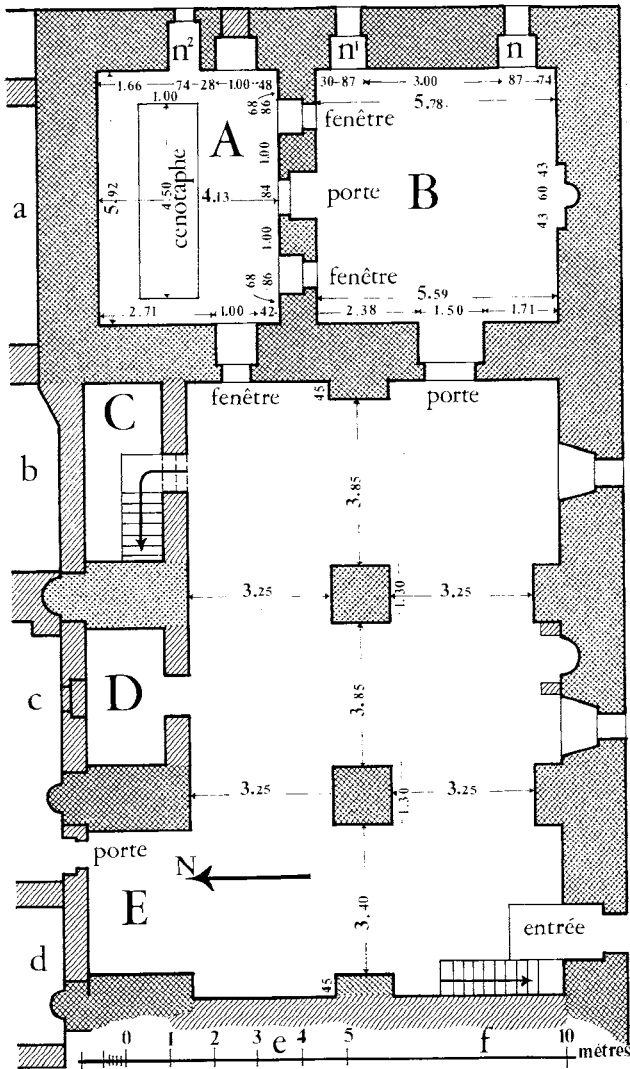
مسقط أفقي
