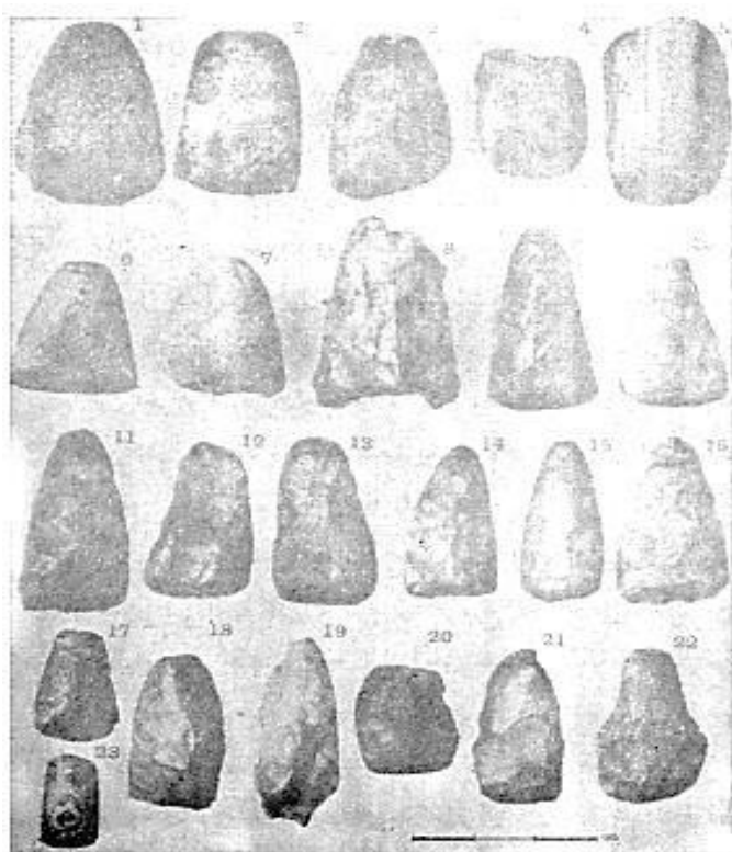
آلات للطحن وبلط من العصر الحجري الحديث.
