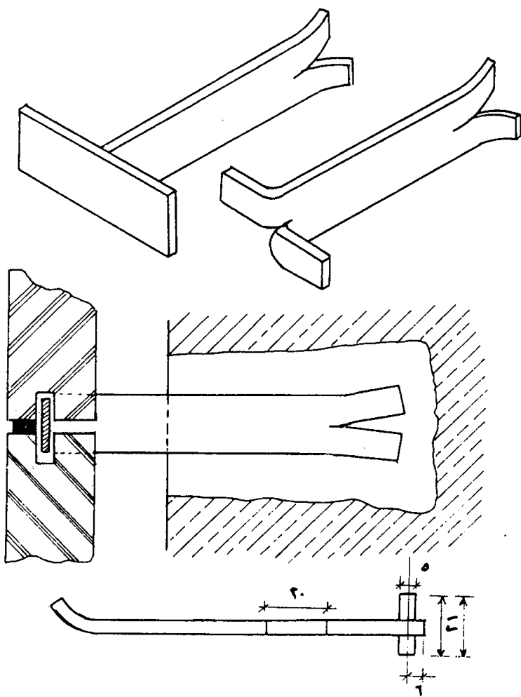
طرق تثبيت الكانات
