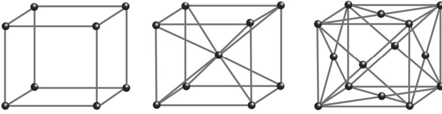
مكعب بسيط
