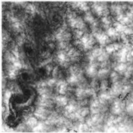
Karman street شارع كارمن
