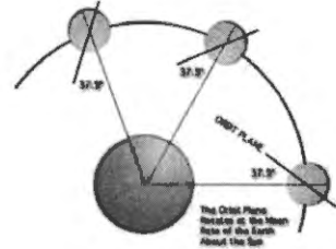
mean sun شمس متوسطة
