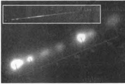
meteor trail أثر نيزك
