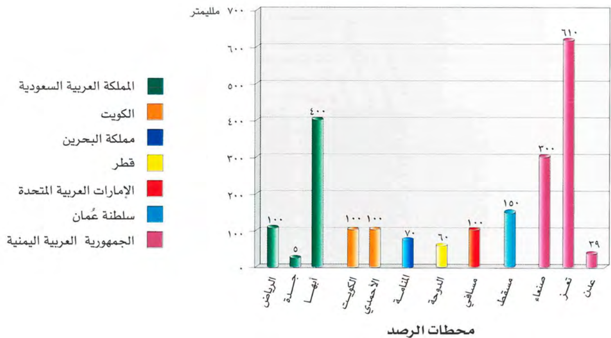
كميات الأمطار السنوية في بعض محطات الرصد لدول شبه الجزيرة العربية
