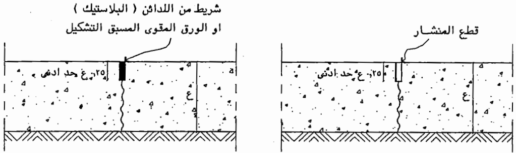
فواصل تحكم ذات مواد مسبقة التشكيل
