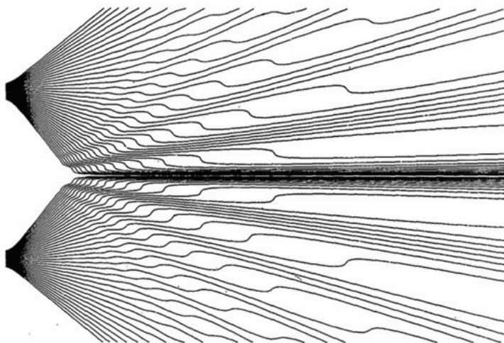
شكل رقم ١٥ مسارات الجسم في تجربة الشقين كما تتنبأ بها نظرية دي برولي - بوم
