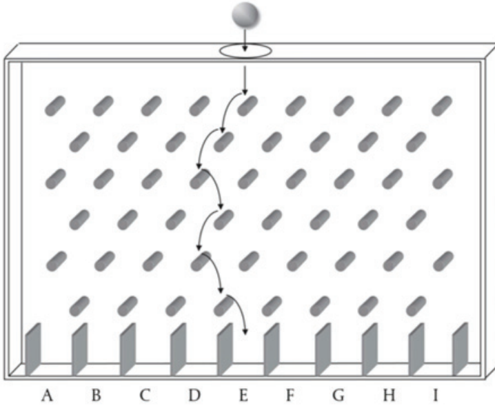
شكل رقم ١١: لوح دبابيس بوبر.
