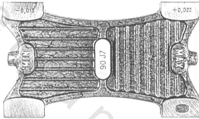
شكل 266 محدد قياس مسطح
