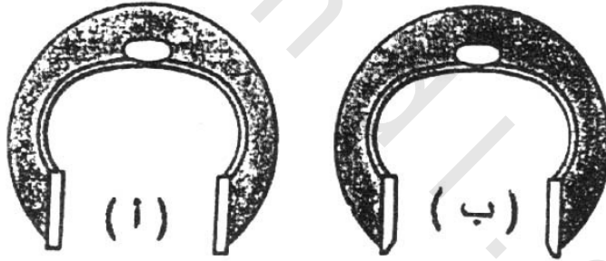
شكل 268 محدّد قياس فكّي أحادي الطرف
