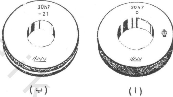
شكل 274 محدد قياس حلقي
