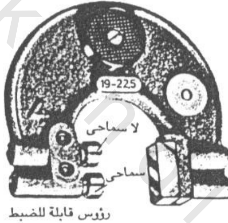
شكل 273 محدد قياس فكي قابل للضبط.
