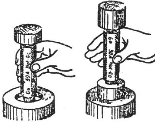
شكل 264 محدد قياس سداي ذو جانبيين ثنائي الطرف أثناء فحص ثقب بالطريقة الصحيحة
