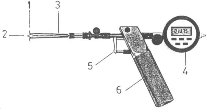
شكس 345 مسدس فحص ثقب الأقطار الصغيرة
