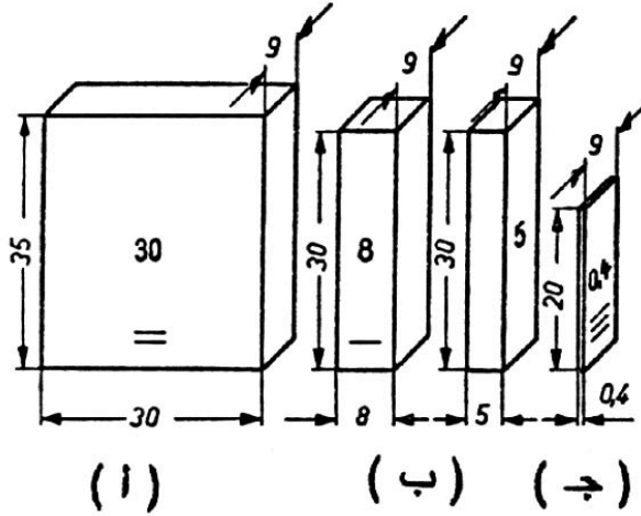
شكل 294 أبعاد قوالب القياس
