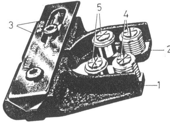
شكل 280 محدد قياس اللولب الفكي القابل للضبط
