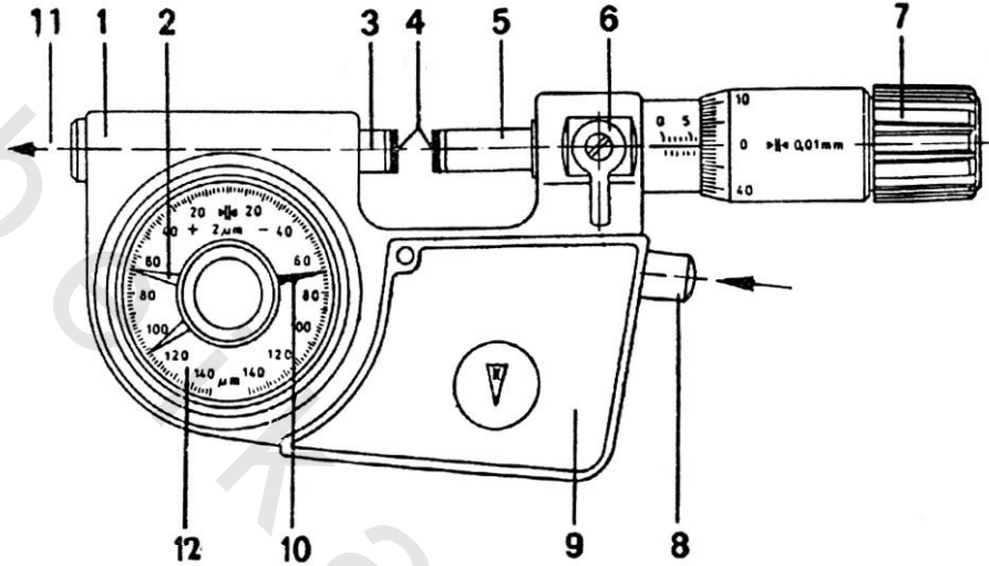
شكيد 332 ميكرومتر البياني الخارجي
