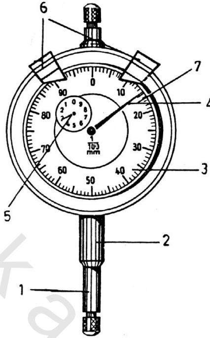
شكل 312 مبين القياس ذو القرص المدرج
