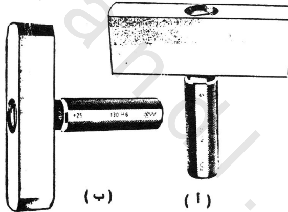
شكل 265 محدد قياس لוחي
