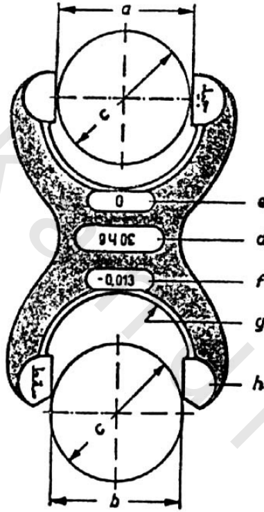
شكل 271 استخدام محددات القياس الفكية المزدوجة للتحقيق من قياس المشغولات بين الحدين الأكبر والأصغر
