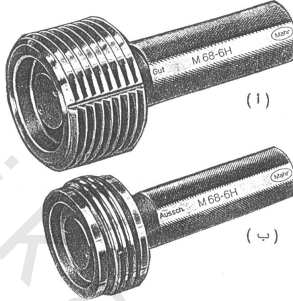
شكل 276 محدد قياس اللولب السدادي أحادي الطرف
