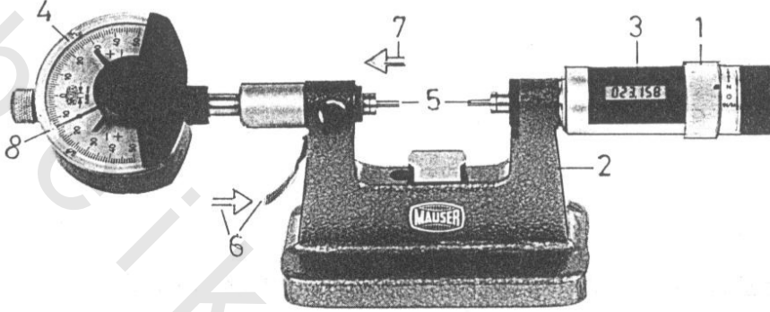
شكل 336 الميكرومتر البياني الخارجي المصمم لعدة أغراض
