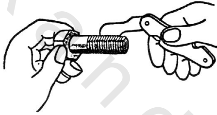
شكل 285 التعرف على خطوة أي لولب ربط وتثبيت باستخدام محدد قياس خطوة القلاووظ
