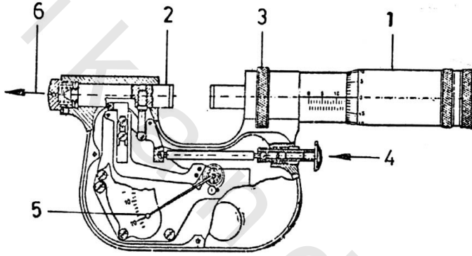
شكس 333 قطاع بالميكرومتر البياني
