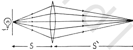
شكل 405 عدسة لامة بين مصدر ضوئي وحاجز
