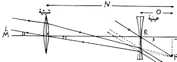
شكل 418 رسم تخطيط لمنظار جاليليو
