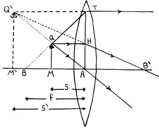
شكل 407 الصورة التقديرية للعدسة المحدبة
