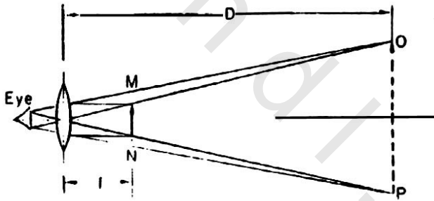
شكل 410 رسم تخطيطي لأساسيات التكبير بمجهر بسيط
