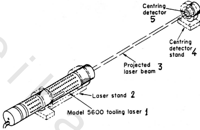
شكل 431 كشاف الليزر المركزي
