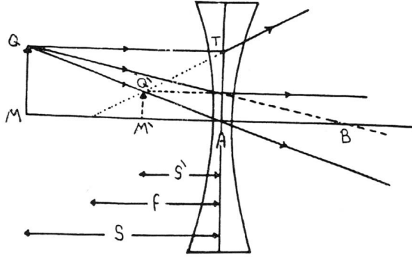
شكل 408 الصورة التقديرية للعدسة المقعرة
