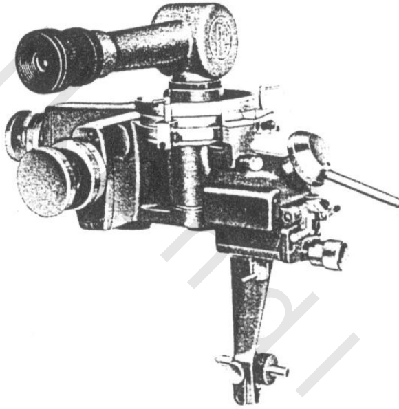
شكل 412 جهاز التحكم البصري
