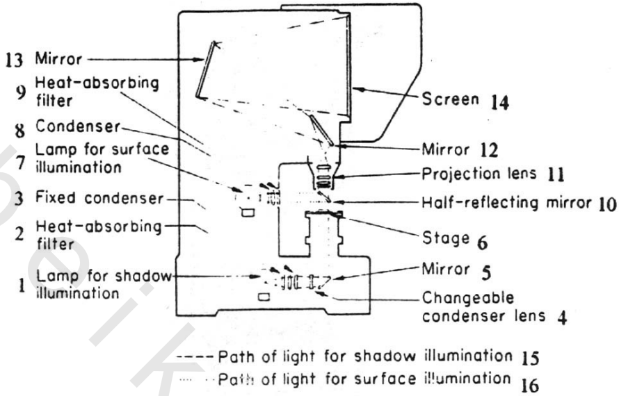
شكل 421 رسم تخطيطي لجهاز الإسقاط البصري
