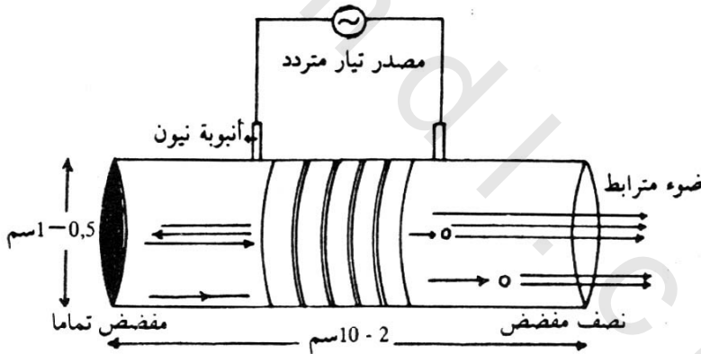
شكل 425 الحصول على الليزر من الأجسام الصلبة
