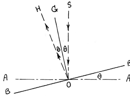
شكل 401 انعكاس الضوء على سطح منحرف
