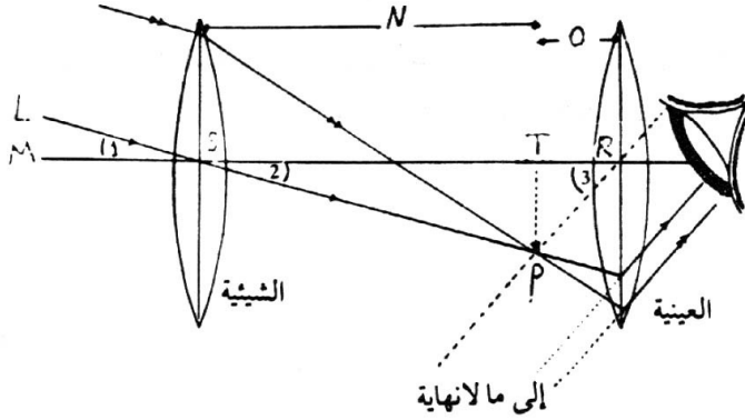
شكل 416 رسم تخطيطي للمنظار (التلسكوب) الفلكي
