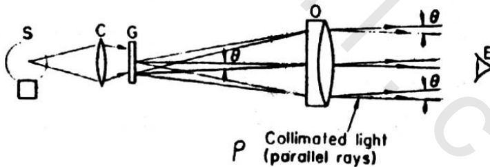
شكل 423 قاعدة أو مبدأ جهاز موجة الأشعة
