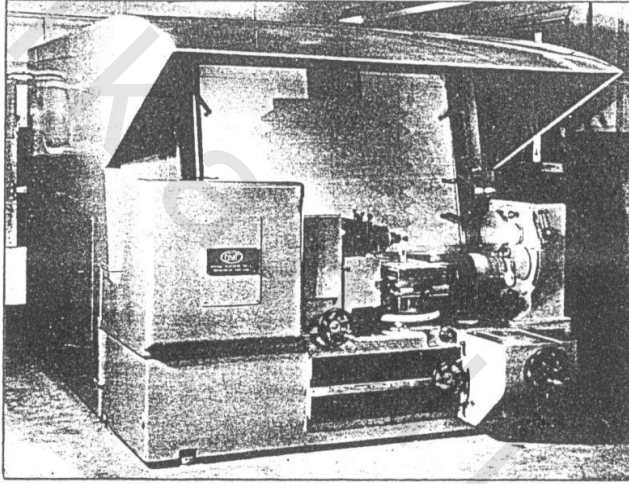
شكل 422 جهاز الإسقاط العام ذو السعة الكبيرة
