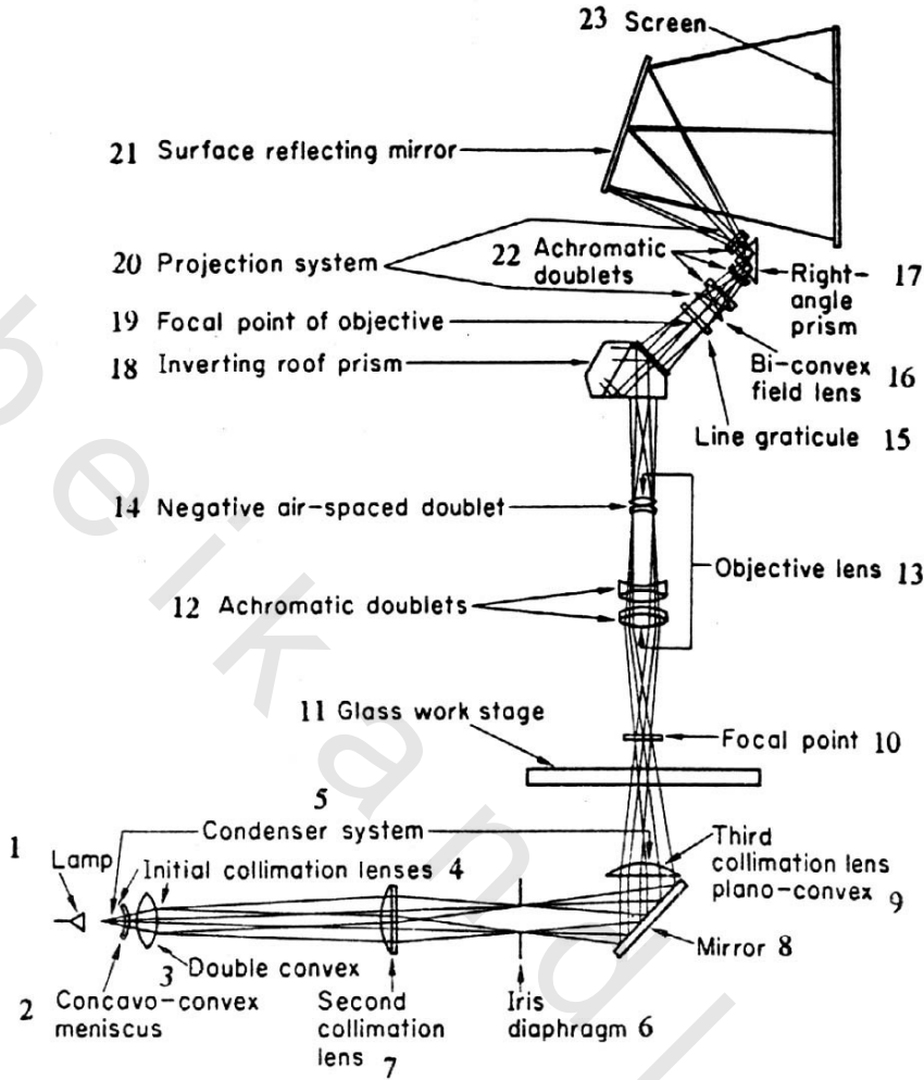
شكل 414 رسم تخطيطي لميكروسكوب صانع الآلة
