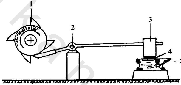
شكل ٤ - ١ المطرقة ذات العجلة المسننة
