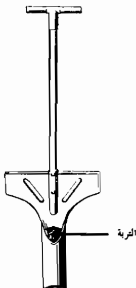
شكل (٨ - ٢) : الـ bulb setter وهى آلة تستعمل فى إحداث ثقب فى الغطاء البلاستيكي ، وحفرة بالتربة لوضع الشتلة .
