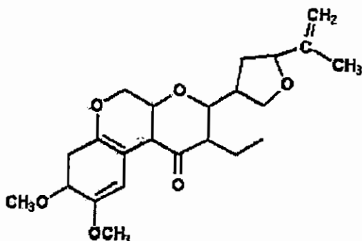
شكل (٤-٢): التركيب البنائى للروتينون.
