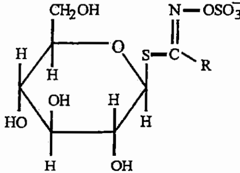
شكل (٢-٢): التركيب الأساسى للجلوكوسينولات glucosinolates.
