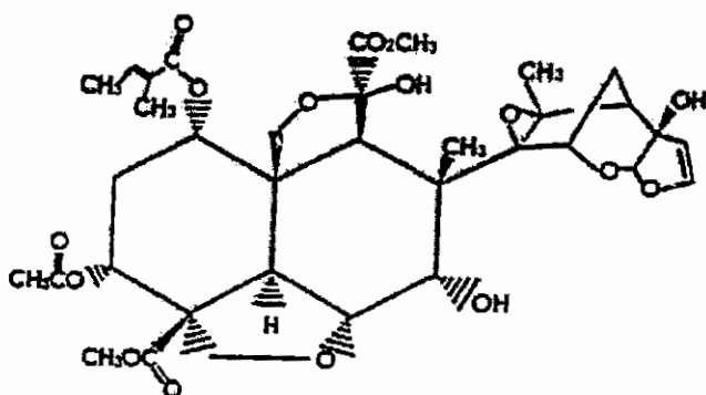
شكل (٤-١): التركيب البنائى للآزاديراكتين Azadirachtin.
