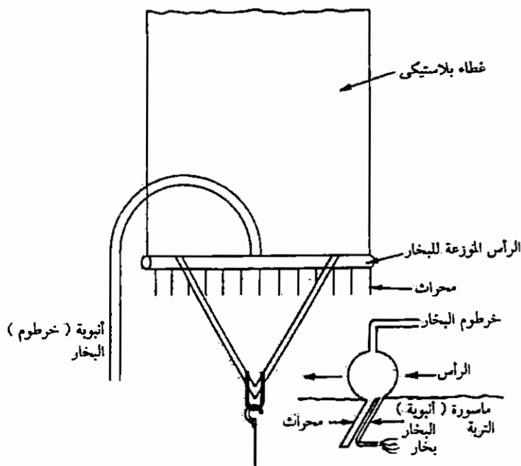
شكل (١-٢): تعقيم تربة الحقل والبيوت المحمية بالبخار (عن Nelson ١٩٨٥).
