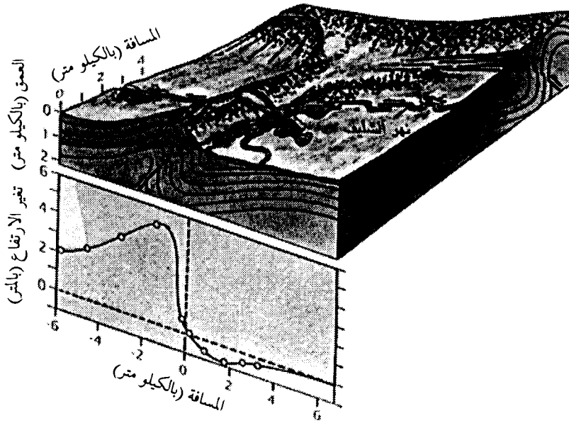
الصورة رقم ٢- مجسم يوضح مرور نهر الشليف في مدينة الأصنام بالجزائر من خلال ممر ضيق عبر الطية في موقع الهزة الأرضية. وكيف ان ارتفاع الأرض خمسة أمتار نتيجة الهزة حج المجرى (المصدر ٨).
