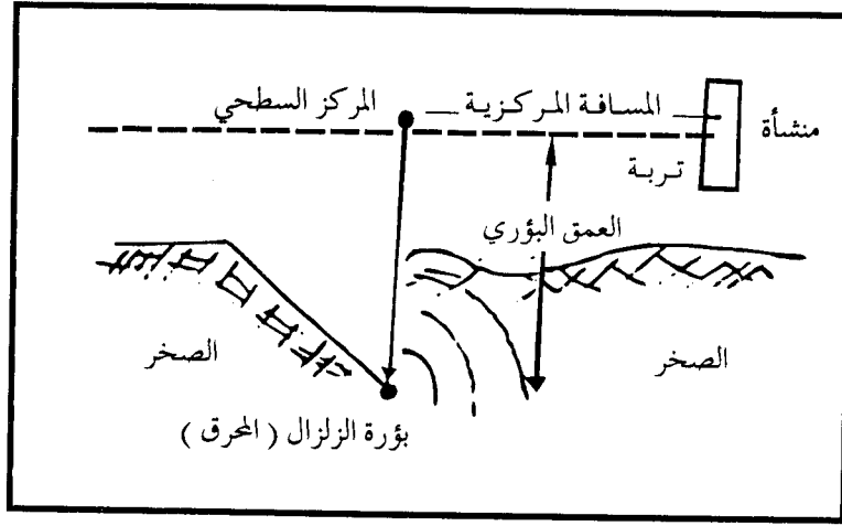
الشكل - ٣٠ - أحداثيات مركز الزلزال (البؤرة)
