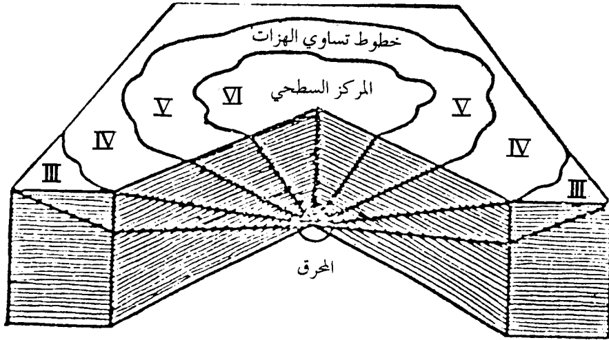
الشكل - ٣١ - شكل فراغي يبين خطوط الشدة المتساوية للهزة الأرضية ومركز الهزة.
