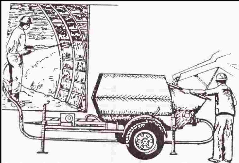
صورة توضح عمل الخرسانة بواسطة مدفع الخرسانة في أحد الأنفاق والتي تصب الخرسانة فيها بدون عمل فرم خشبية لها كذلك تستخدم هذا النوع من الصب في أعمال لترميمات والقمصان SPRAYED CONCRETE BY CEMENT GUN & SHOUTCRE
