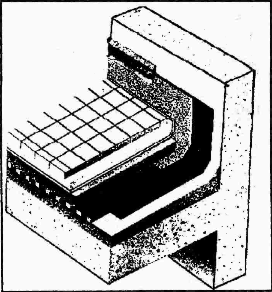
قطاع عزل حراري للأسطح بواسطة الأسْتِروْبور
