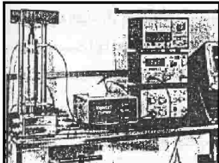
جهاز الالتراسونيك ULTRA SONIC CONCRETE TEST
