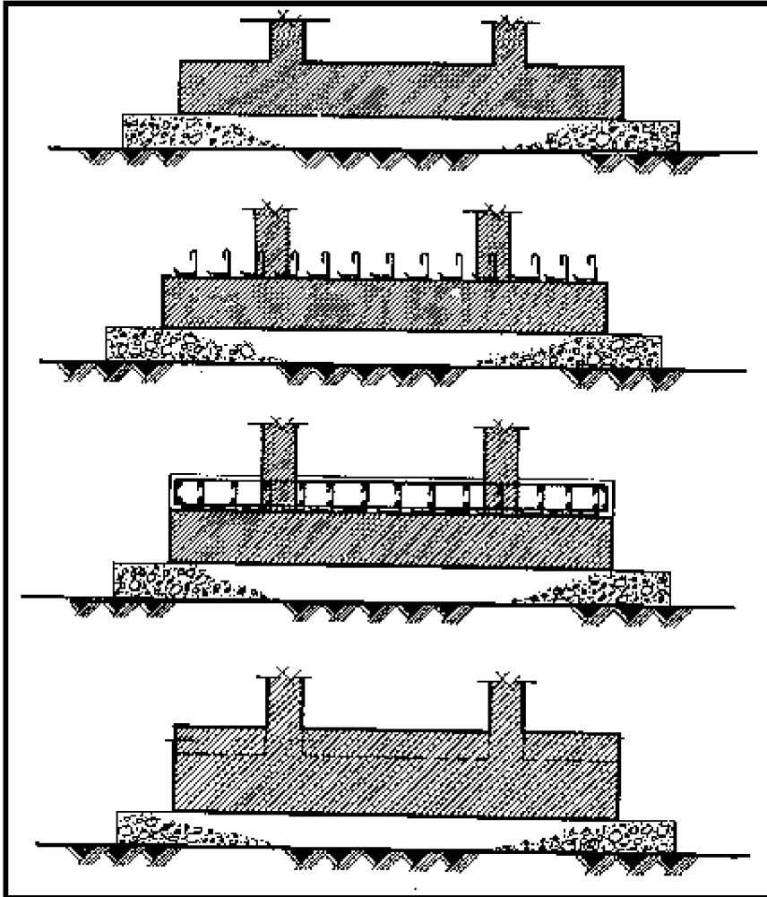
طريقة زيادة قطاعات الأساسات
