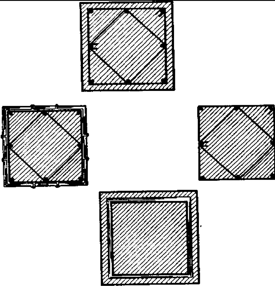
تقوية وعلاج الأعمدة بتثبيت زوايا وألواح حديدية حول العمود
