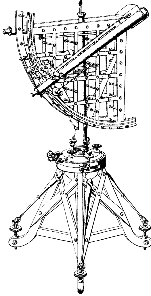
ربعية محمولة يعود تاريخها إلى مطلع القرن التاسع عشر. من بيرسون (1824). المصدر: مكتبة وولباخ، جامعة هارفرد.
