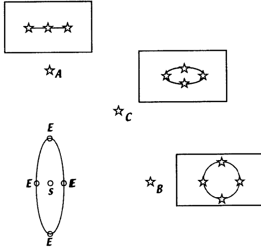
حركة اختلافات المنظر السنوية في مواقع مختلفة من مدار الأرض.
