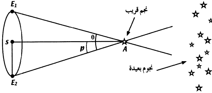
اختلاف منظر نجم
