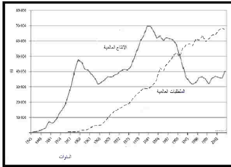
الشكل ٢. مفاعل اليورانيوم في العالم، ومتطلبات الانتاج من المناجم، ١٩٤٥-٢٠٠٤ (١) Figure 2. World Uranium Reactor Requirements and Production from Mines, 1945–2004
