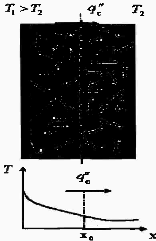
الشكل (1 - 2) انتقال الحرارة بالتوصيل
