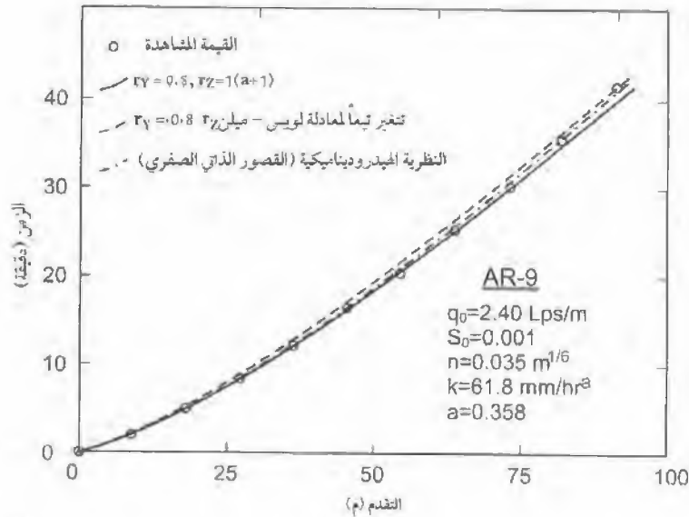
الشكل رقم (١٣, ١). مقارنة بين النظرية والتجربة في الشريحة على التدرج المتوسط.
