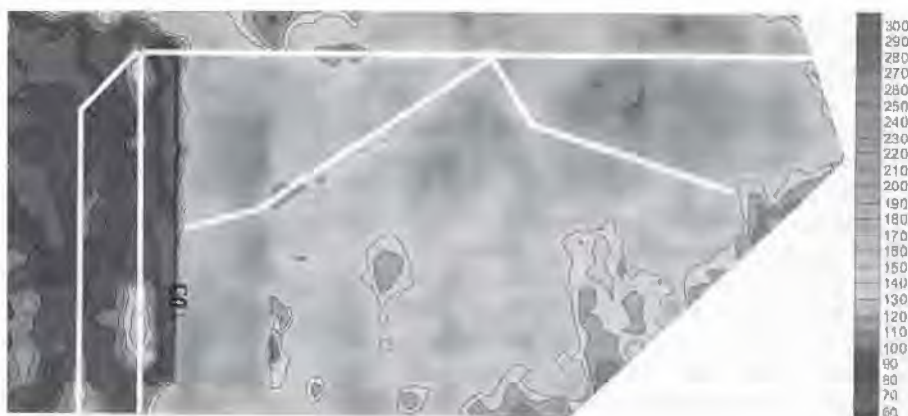
الشكل رقم (١٨, ١٤). مسح EM38 للمراعي المروية بعد ثلاث سنوات من تركيب نظام الصرف تحت السطحي والذي يوضح معامل التوصيل الكهربائي الظاهري للتربة ( EC_a ). الخطوط البيضاء هي أنابيب نظام الصرف تحت السطحي (Christen et al. , 2004).
