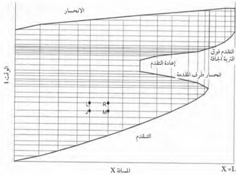
الشكل رقم (١٣,٧). شبكة الحساب في المستوى x-t .
