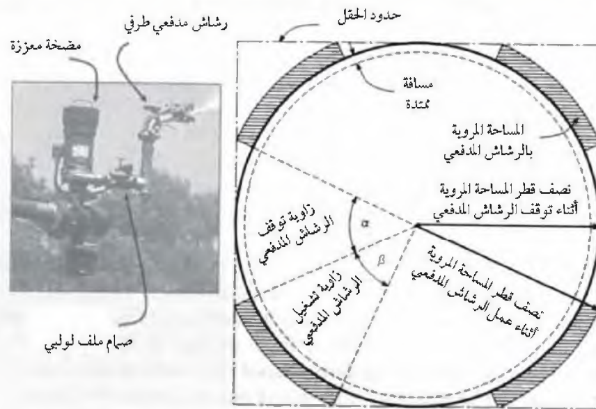
الشكل رقم (١٦، ٢٠). مكونات وتخطيط حقل لنظم الري ااخورية النمطية.
