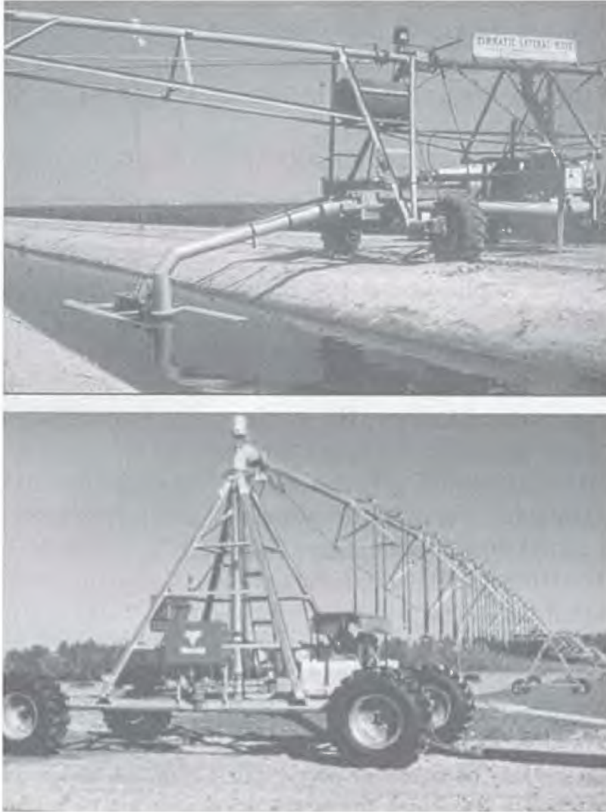
الشكل رقم (١٦,٣٢). أمثلة على نظم الحركة المستقيمة التي يتم إمدادها بنظام قناة وعمرطوم قابل.
