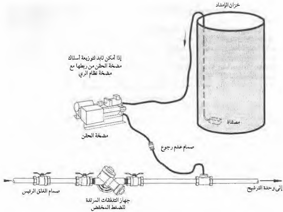
الشكل رقم (١٩, ١). مخطط نموذجي لأنظمة مضخات الحقن ذات الإزاحة الموجبة (van der Gulik, 1993).
