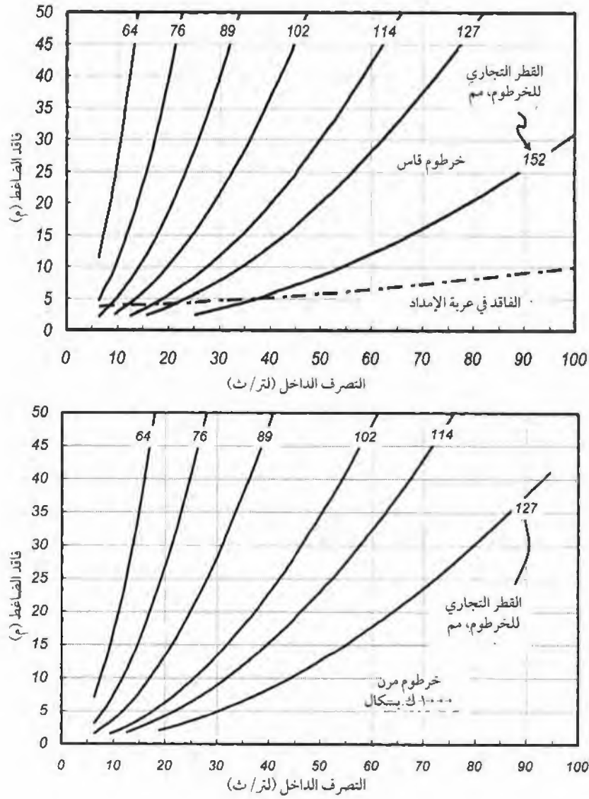
الشكل رقم (١٦, ٣٣). فاقد الضاغط في الخراطيم القاسية والمرنة في نظام الحركة المستقيمة ونظم الري المتقلبة. وموضح كذلك فاقد الضاغط في عربة الإمداد بالنسبة للناقلات.
