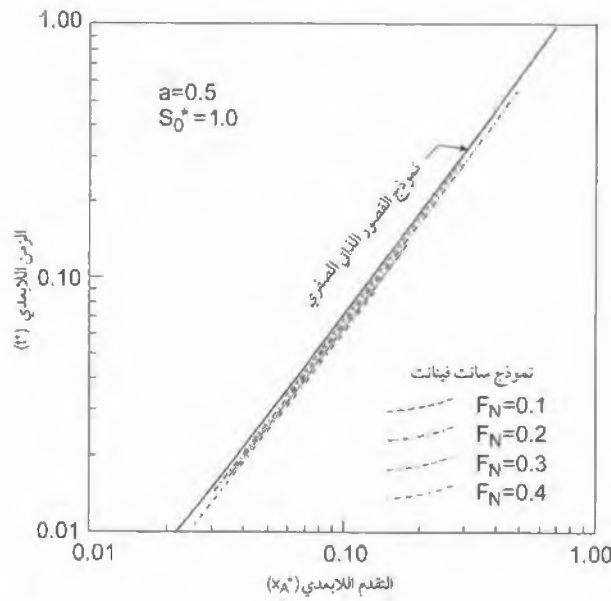
الشكل رقم (١٣, ١٠). تأثير رقم فروود المرجعي على تقدم مجرى التيار.
