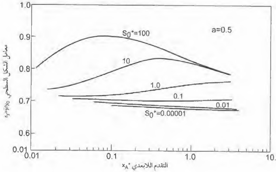
الشكل رقم (١٣, ١٤). تقييم معامل شكل المجرى المائي السطحي كدالة في ميل العمق النسبي.
