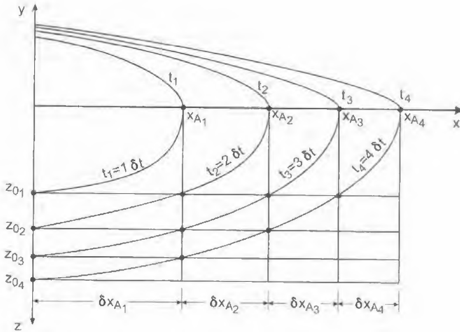
الشكل رقم (١٣, ٣). التسرب التراكمي أثناء التقدم. ويتم الفصل بين خطوط الزمن بالثابت \delta t .
