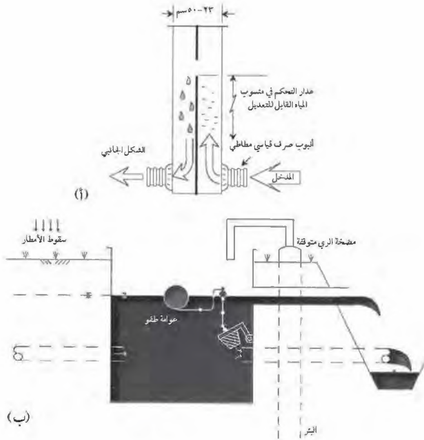
الشكل رقم (١٨,٣). (أ) جهاز تحديد التدفق من نوع الهدار داخل أنبوب صرف أو أنبوب رفع فرعية، و(ب) صمام التحكم في التدفق الذي ينشط بالطفو داخل أنبوب صرف أو أنبوب رفع فرعية.
