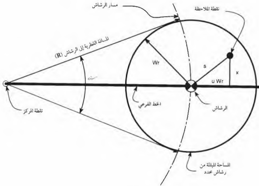
الشكل رقم (١٦،٢٥). توضيح للمعاملات المستخدمة في حساب النظامية إضافة المياه في نظم الري المحورية.
