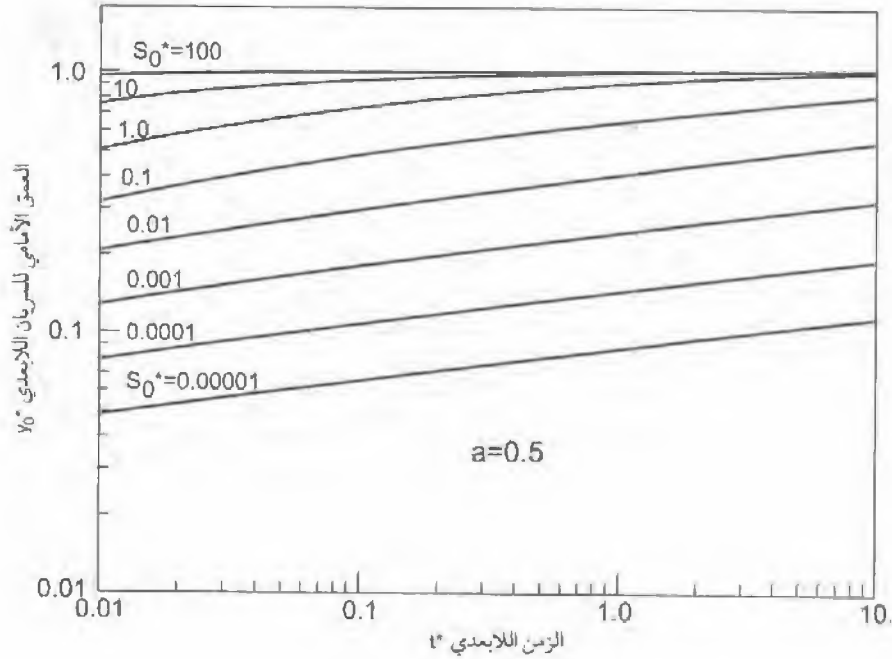
الشكل رقم (١٣,١٣). زيادة العمق الأمامي للسريان كدالة في الميل النسبي للقطاع.
