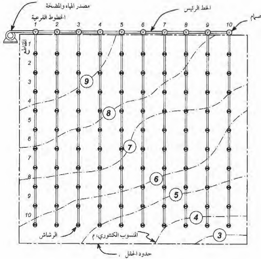
الشكل رقم (١٤, ١٦). منظر مسطح لحقل مروي باستخدام نظام الرش الثابت.
