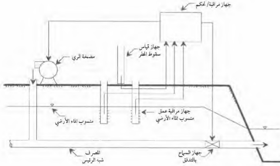
الشكل رقم (١٨،٥). رسم تخطيطي لتحكم التغذية الاسترجاعية الآلي لتصريف الري التلقائي بالجاذبية.
