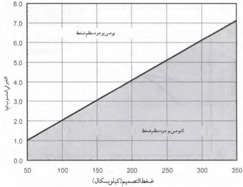
الشكل رقم (١٥،٦). التغير في النسوب المناظر لتغير قدره ٢٠٪ في ضغط التصميم.
