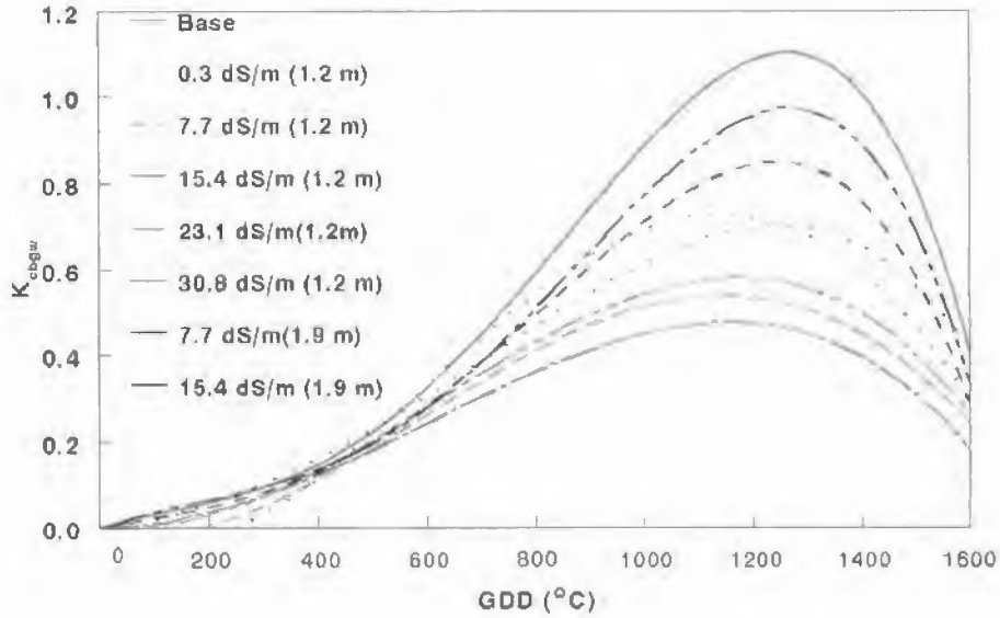
الشكل رقم (١٨،٧). معامل باسال محصول القطن والمحسارات معاملات المحصول المعدلة المشتقة من بيانات الليسوميترات لخمس كميات من المياه الجوفية عند أعماق مختلفة.
