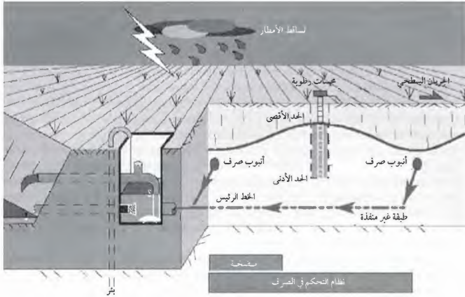
الشكل رقم (١٨، ١). نموذج للتحكم في الصرف والري التحقي عند تشغيل إدارة منسوب الماء الأرضي، التحكم في مستوى مصب المياه (غرفة التفريغ) يعتمد على التغذية الراجعة لعمق منسوب الماء الأرضي في الحقل.
