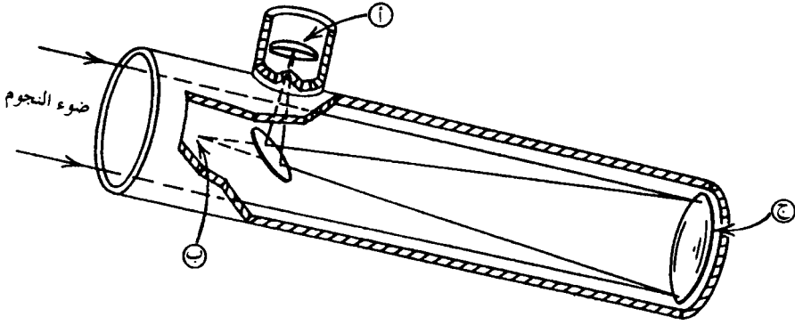
الشكل 8.2 رسم لمقرب نيوتن العاكس يُظهر مرآته الرئيسية، ومرآته الثانوية الصغيرة المنحرفة، وعدسته العين.
