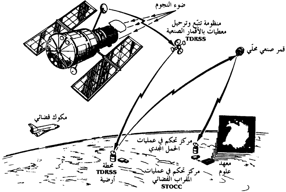
الشكل 13.2 مسار المعطيات التي بينها مقراب هبل Hubble الفضائي.
