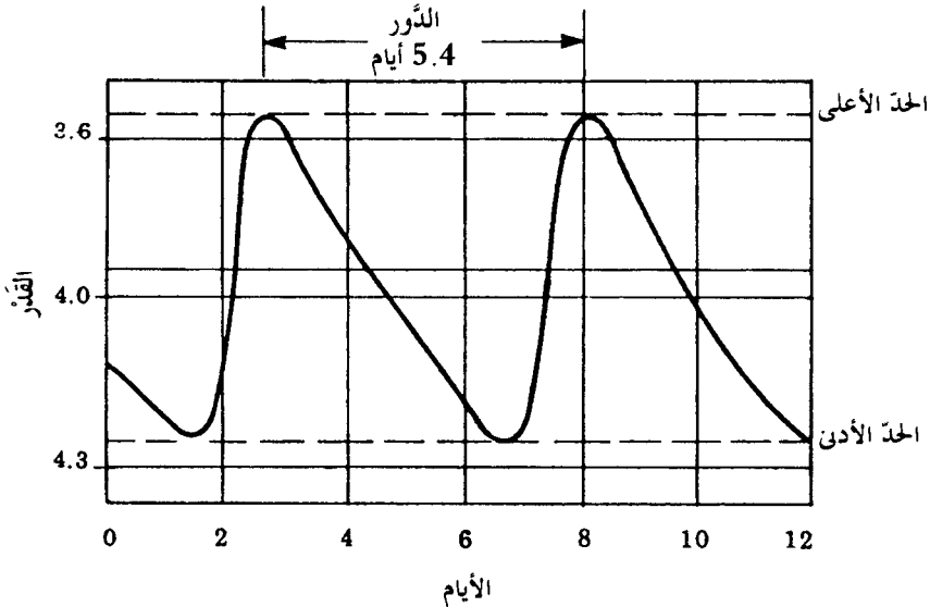
الشكل 7.5 منحني الضوء، يُظهر تغيّر خُرْج الضوء للمتغيّر القيفاوي الأولي دلتا قيفاوس.
