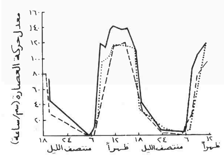
الشكل رقم (٥-١٦). التغير الدوري لمعدل حركة العصارة لثلاثة أنواع نباتية (____) Picea و Larix, (-----) و (.....) Fagus.
