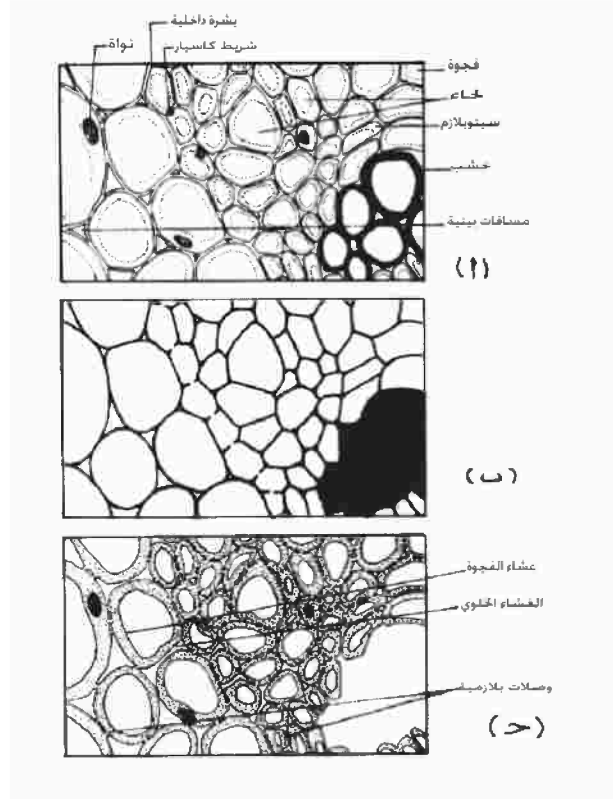
الشكل رقم (٥-٨). أ-رسوم تخطيطية لجزء من قطاع عرضي في جذر نبات الشقيق. ب-الأجزاء الميتة من الخلايا (Apoplast) باللون الأسود، و ج-الأجزاء الحية من الخلايا (Symplast) بالأجزاء المنقطة.
