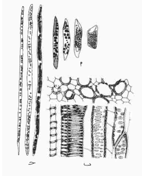
الشكل رقم (٥-١٣). رسم توضيحي لعناصر الخشب. أ- أشكال الأوعية الخشبية بعد فصلها من النسيج. ب- منظران للأوعية الخشبية في قطاع عرضي والأوعية في وضع رأسي. ج- القصبيات.
