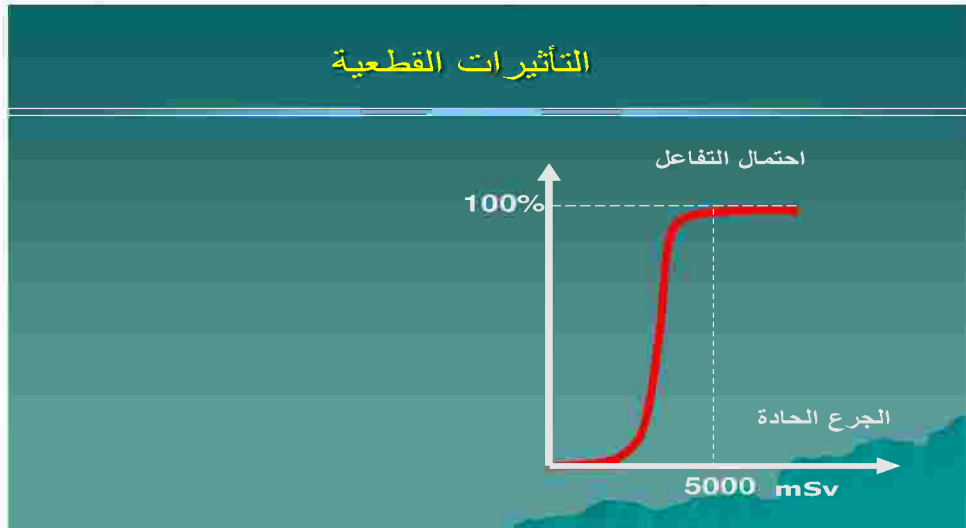
شكل ( ٢ - ٧ ) التأثيرات القطعية للإشعاع واعتمادها على جرعة العتبة
