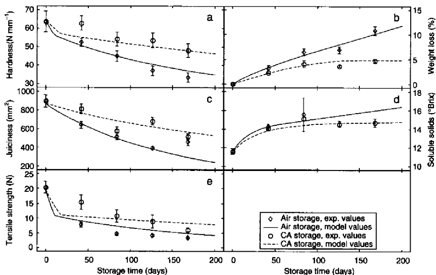
الشكل رقم (٩,٥). التغير في نواتج المتغيرات المقاسة أثناء التخزين. ترمز أعمدة الخطأ إلى فترات الثقة ٩٥٪ لم توسط ٢٠ قياساً (لاحظ أن قيمة المواد الصلبة الذائبة بعد ٨٤ يوماً في التخزين في الهواء هي متوسط فقط لثلاث قياسات) (أعيد النشر من قبل دي اسميث، ٢٠٠٠) مع إذن خاص من السيفر ساينس Elsevier Science.
