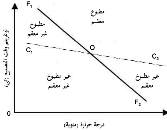
الشكل رقم (٦، ١٠). علاقة التي - التي t-T للتحميم الميكروبي، إف (F)، والطبخ، سي (C)
