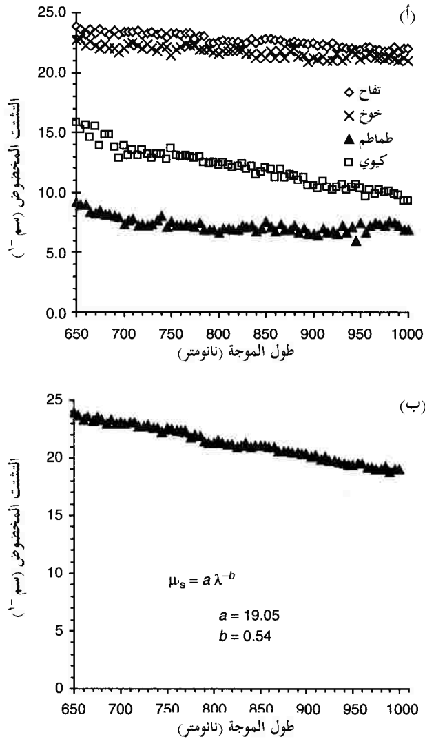
الشكل رقم (٨,٨). (أ) طيف التشتت للتفاح والخوخ والطماطم وفاكهة الكيوي (ب) أفضل ملائمة ومطابقة لنظرية ميلي لطيف التشتت لتفاح الاستار كينج.
