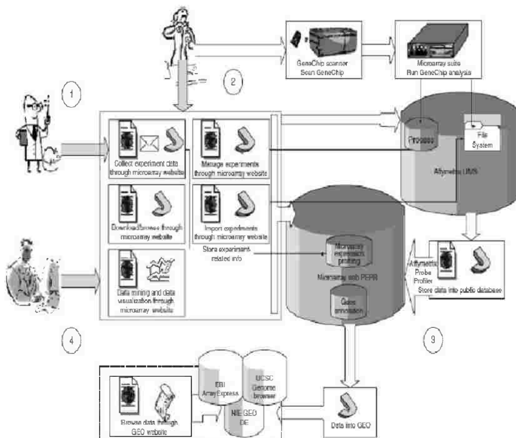
الشكل رقم (١١، ١٢) تصميم هيكل لموارد تعريف التعبير العام PEPR . من http://pepr.cnmcresearch.org .
