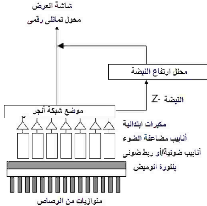
الشكل رقم (١،٦) شكل تخطيطي لكاميرا أنجر لأشعة جاما المستخدمة في الطب النووي المستوى.
