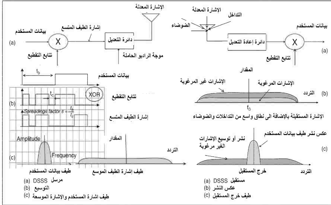
الشكل رقم (٨، ١٠) التراسل بالطيف المتسع.
