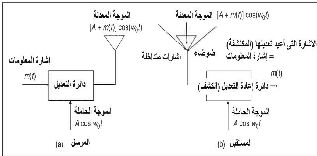
الشكل رقم (١٠،٧) التراسل بموجات الراديو الضيقة النطاق.
