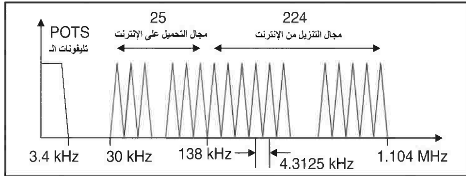
الشكل رقم (١٠,١) الطيف الترددي لل ADSL.
