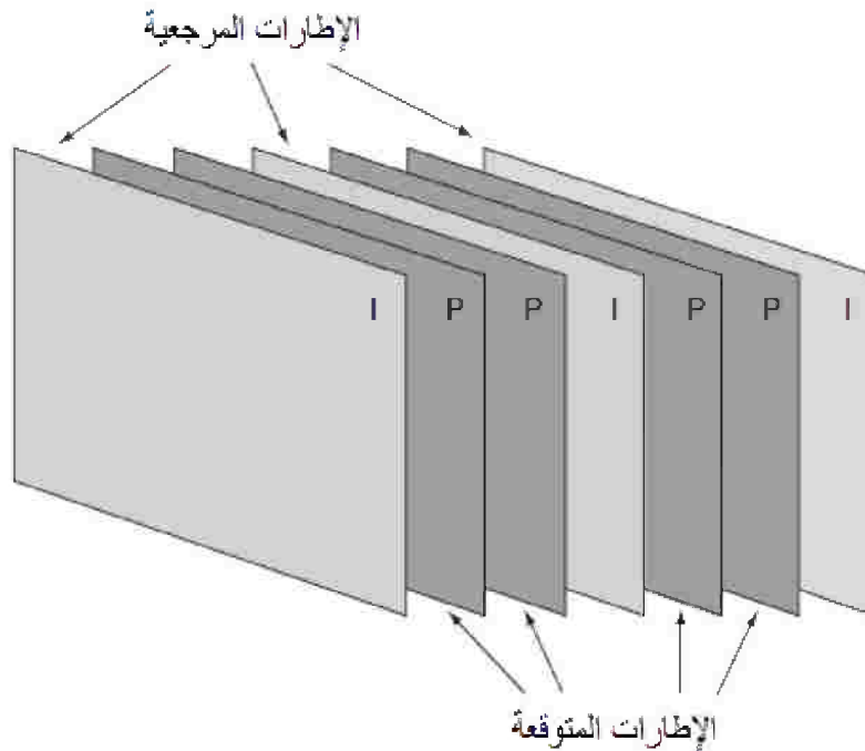
الشكل رقم (٣،١٥) ترتيب الإطارات المرجعية (I) والفرقية (P) لتشفير الفيديو المجهن.
