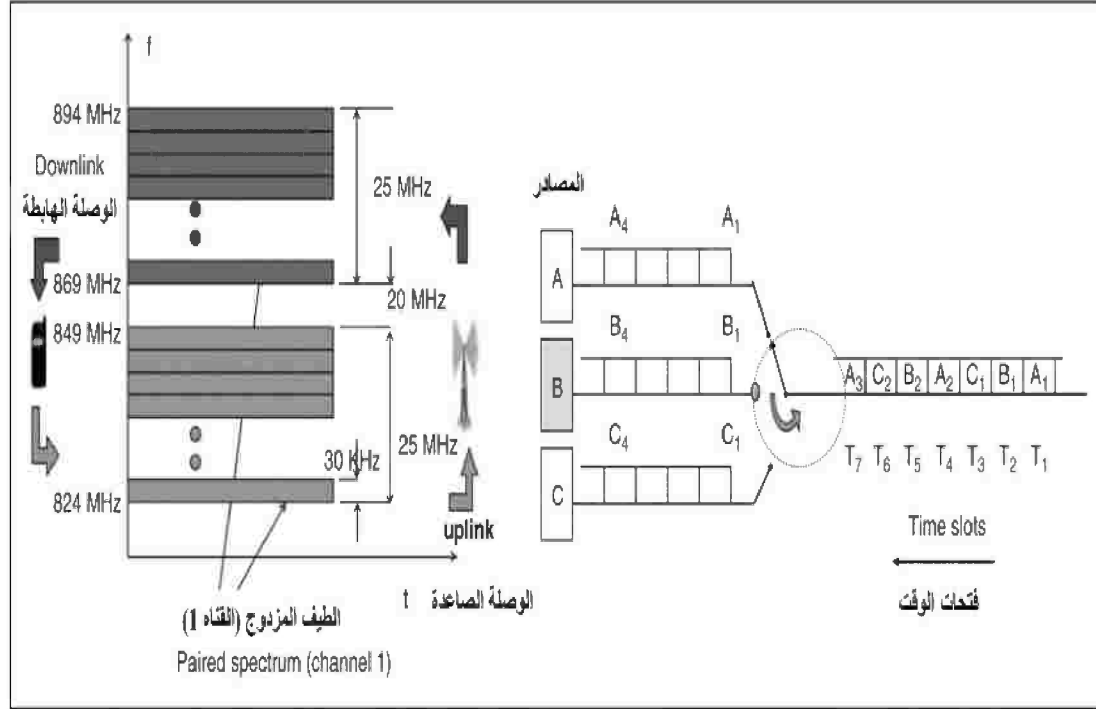
الشكل رقم (١٠،٢) طرق الاتصال المتعدد
