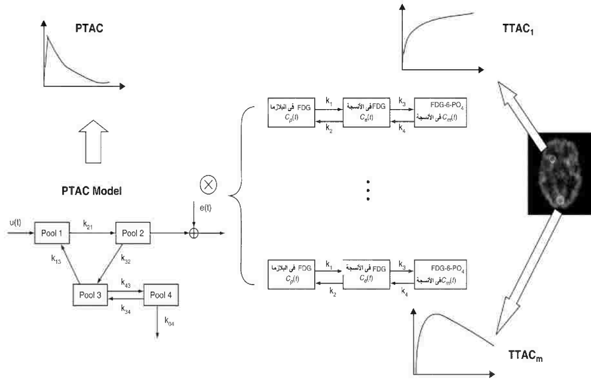
الشكل رقم (٦،١١) مخطط سير للنمذجة المتتالية لطريقة التخمين المتزمن حيث \otimes هي عملية الضرب الالتفافي.
