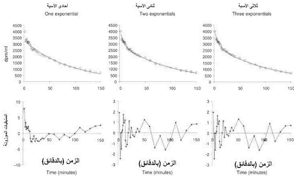
الشكل رقم (٥،٨) أحسن موائمة للبيانات المعطاة في الجدول رقم (٥،١) للنماذج أحادية وثنائية وثلاثية الأسية مع رسم المتبقيات الموزونة في كل حالة. المعاملات الأسية والقيم المميزة لكل نموذج معطاة في الجدول رقم (٥،٢).
