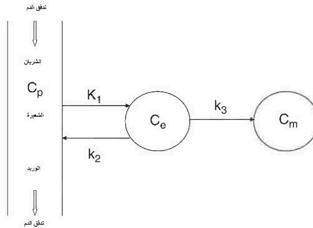
الشكل رقم (٥.١٠) نموذج الحجيرة النسيجي الثنائي.
