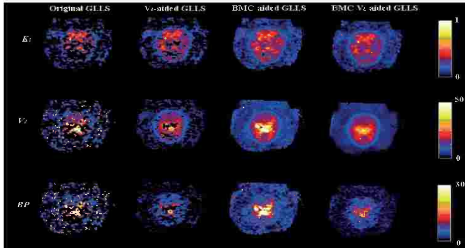
الشكل رقم (٦،٢٠) الصور البارامترية لمعدل التدفق الداخل ، K_1 ، والتوزيع الحجمي : V_d = K_1/k_2(1+k_3/k_4) ، واحتمال الترابط BP = K_1k_3/k_2k_4 . قيم الفوكسيل والتي ليس لها توقعات معدل ثابت. (معدل ثابت سالب أو أكبر من الواحد) تم وضعها تساوى صفراً.
