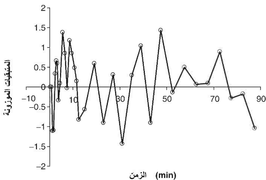
الشكل رقم (٥,٦) رسم المتغيرات الموزونة في مقابل الزمن.
