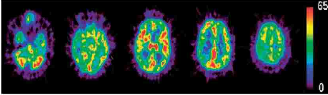
الشكل رقم (٦،١٣) صور ال rCBF باستخدام دالة الدخل المستنتجة بالصورة من دراسات ال 150-water.
