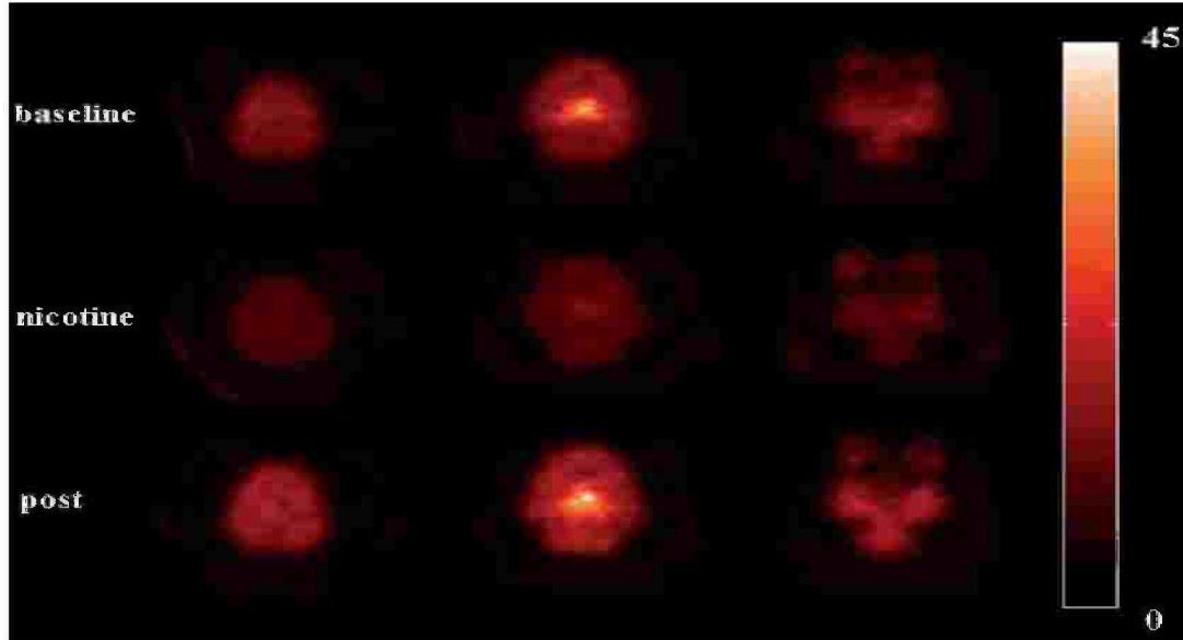
الشكل رقم (٦،١٩) الصور البارامترية لل V_d لحالة الخط القاعدي، وغرس النيكوتين ، وبعد حقن النيكوتين على التوالي. الصور الوسطى في كل صف تبين الوضع الطبيعي ، والانسداد ، وزيادة تنظيم لل nAChRs على التوالي. للحصول على معلومات أكثر
