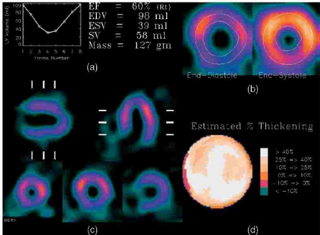
الشكل رقم (٦،١٤). عرض ال SPECT من خلال بوابة باستخدام المعاملات المكعبة الآلية (b). منحنى الزمن الحجمي للبطين الأيسر على مدى دورة قلبية (a)، التغيرات المتوقعة في سمك العضلة (d). لمزيد من المعلومات عن
