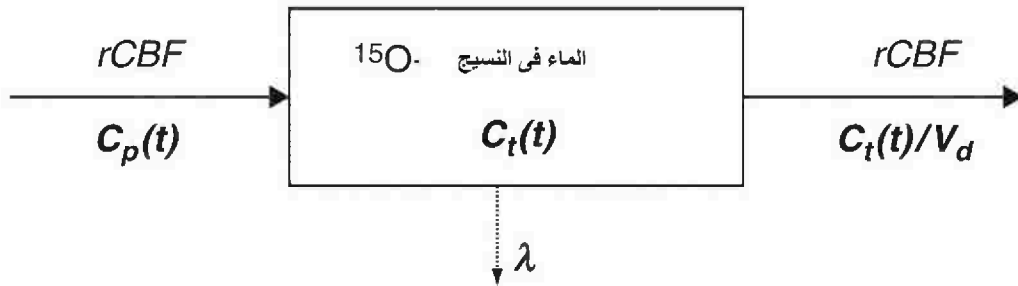
الشكل رقم (٦,٥) نموذج الحجيرة الواحدة لتدفق الدم المخي الموضعي rCBF150 الماء في النسيج.
