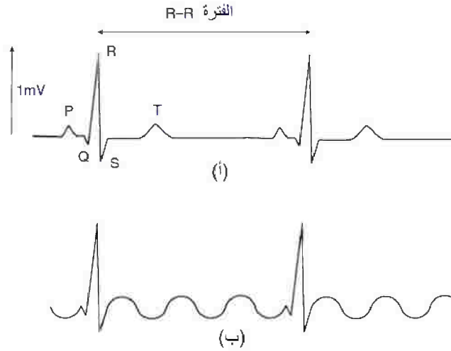
الشكل رقم (١.٢٢) (أ) مخطط كهربى للقلب ECG لشخص سليم. (ب) شكل يبين الرفرفة الأذينية حيث تسافر النبضات التنظيمية في مسقط دائري خلال الأذين.
