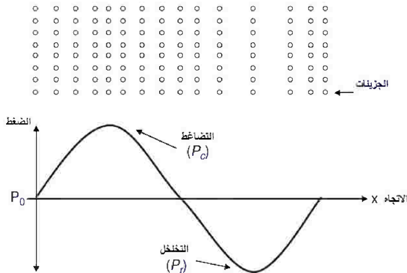
الشكل رقم (١،٩) شكل توضيحي لحركة الجزيئات داخل النسيج نتيجة حركة موجة فوق صوتية.
