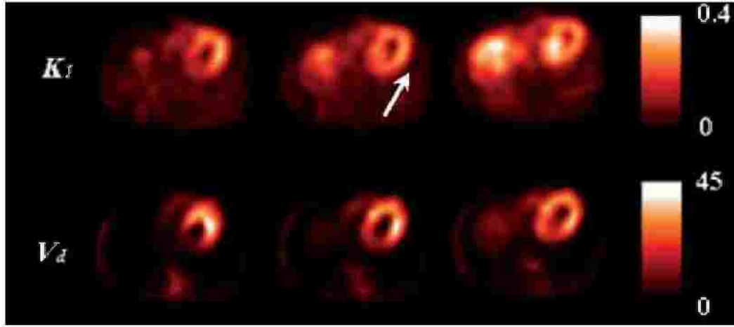
الشكل رقم (٦،١٥) الصور البارامترية ل K1 (a) و Vd (b) باستخدام رسم يوكوى مع 201TI. للحصول على معلومات أكثر.
