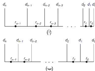
الشكل رقم (٣، ١٣) التكميم القياسي غير المنتظم (أ) والمنتظم (ب). كل مجموعة من مستويات القرار d تقابل استجابة كمية r . بالنسبة للتكميم المنتظم، تكون مستويات التكميم متساوية البعد بين بعضها. في التكميم غير المنتظم تكون المسافة بين مستويات القرار متغيرة.
