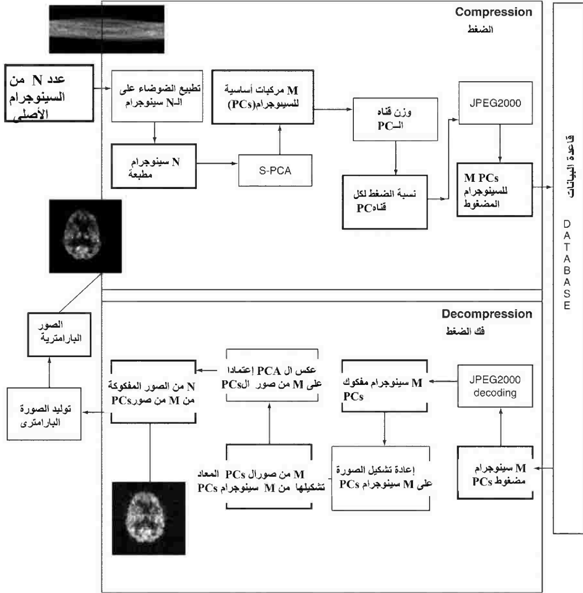
الشكل رقم (٣،٢٢) ضغط بيانات الصور الوظيفية الديناميكية باستخدام PCA والـ JPEG2000 الموزون بالقناة في نطاق السينوجرام
