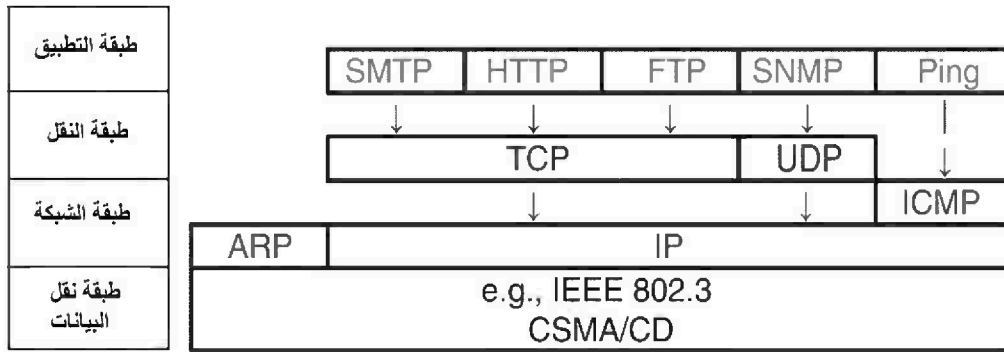
الشكل رقم (٤، ١٠) جزء من طبقات بروتوكول TCP/IP.
