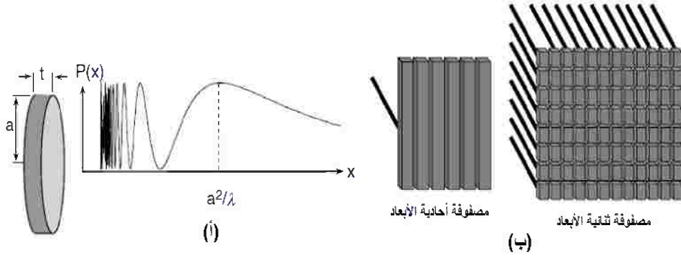
الشكل رقم (١،١١) (أ) رسم توضيحي للموجة الضغطية الناتجة من حساس فوق صوتي في صورة قرص مسطح من عنصر واحد كدالة في المسافة. (ب) رسم تخطيطي لمصفوفات من العناصر أحادية وثنائية الأبعاد.
