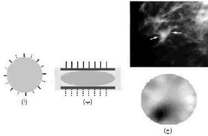
الشكل رقم (١،٢٠) (أ) تضاريس المصدر الضوئي (المتصل) والكاشف (المنقط) في تجربة حقيقية للتصوير الندي (ب) الندي وقد تم وضعه بين لوحين بحيث تم تثبيت المصادر والكواشف (يمكن استخدام سائل للتوافق الضوئي لتحسين التلامس الضوئي) (ج) صورة ال DOT (الأسفل) بالمقارنة بصورة الندي باستخدام الرنين المغناطيسي (أعلى). (S. Nioka, (B. Chance, Technology in cancer research and treatment, vol. 4, pp. 497, 2005
