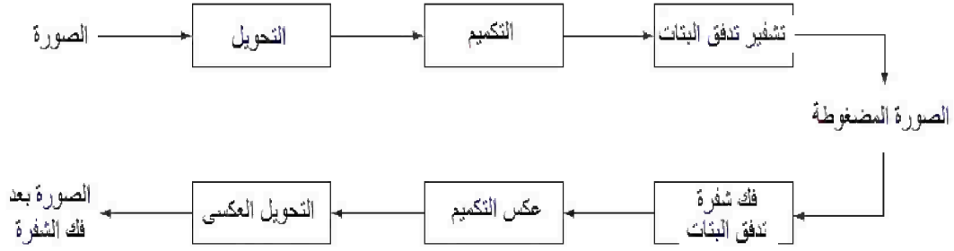
الشكل رقم (٣،٩) المكونات الأساسية لهيكل التشفير المعتمد على التحويل.
