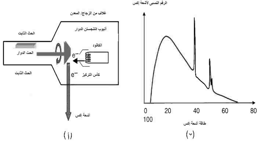
الشكل رقم (١،١) (أ) شكل تخطيطي لأنبوبة أشعة إكس (ب) طيف طاقة مثالي من أنود التنجستين باستخدام جهد تعجيل حوالي ١٠٠ كيلوفولت.
