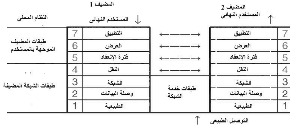
الشكل رقم (٣، ١٠) هيكل السبع طبقات OSI RM.
