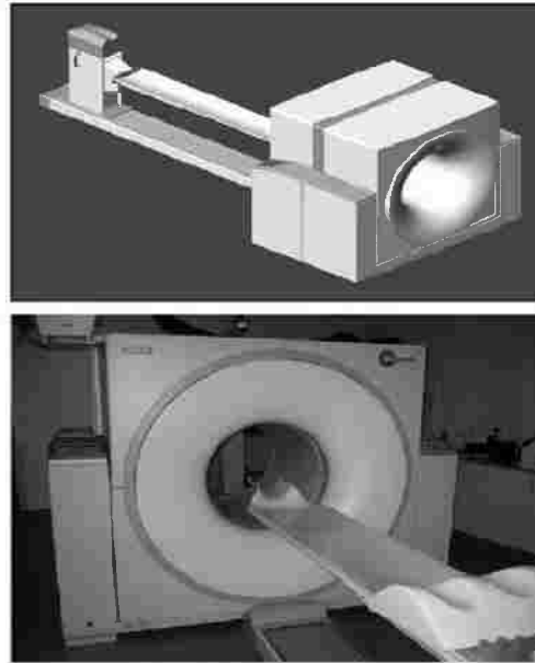
الشكل رقم (٨،٤) صورة تخطيطية وصورة حقيقية لنظام PET/CT تجارى. لقد تم دمج جهاز CT متعدد الشرائح مع نظام PET متقدم من النوع الدوار لتكوين جهاز مهجن من الاثنين. يتم تثبيت ال CT أمام وحدة ال PET. يُمكن فصل هذه الوحدات منفصلة لغرض الصيانة.
