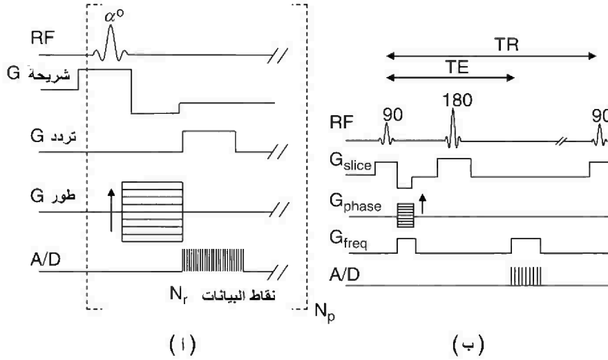
الشكل رقم (١٥,١) (أ) الصدى التدرجي لتتابع الصورة. (ب) الصدى المغزلي لتتابع الصورة.
