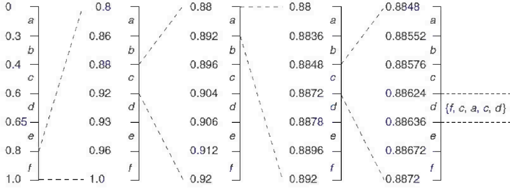
الشكل رقم (٣،٣) التشفير الحسابي مع الفترات المتتالية للرموز {f, c, a, c, d} من التوزيع الإحتمالي في الجدول رقم (٣،١) .
