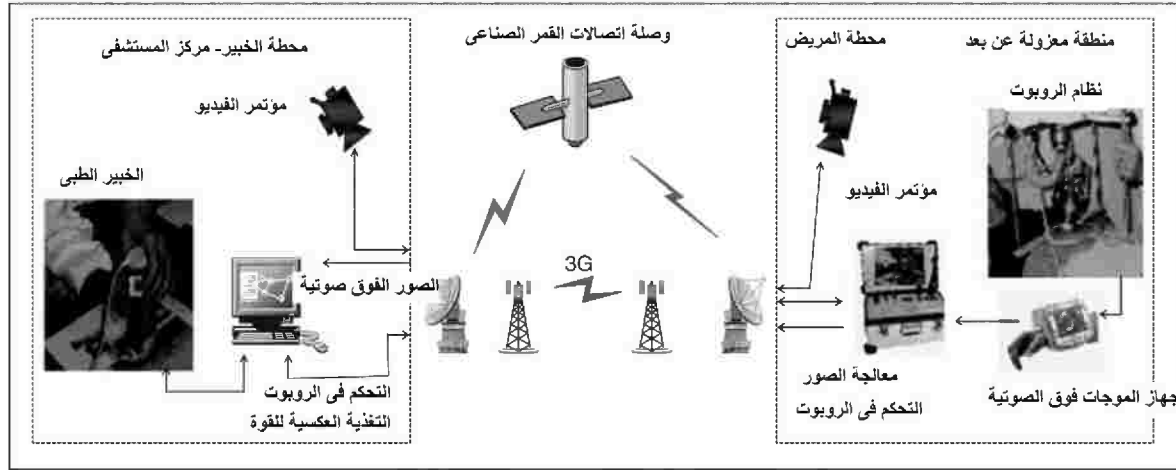
الشكل رقم (١٠،١١) نظرة وظيفية عامة على نظام OTELLO تم الحصول عليها من [29] Garawi et al.
