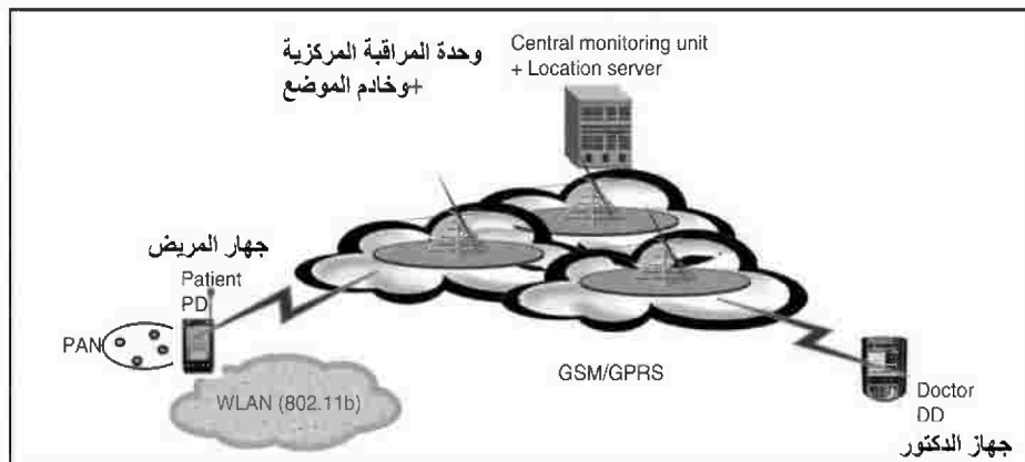
الشكل رقم (١٠،١٠) نظرة عامة على هيكل النظام EmerLoc.
