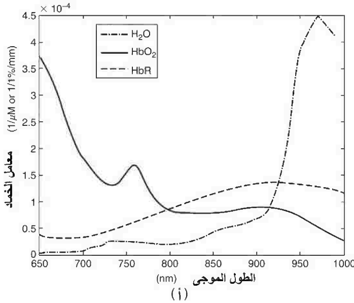
الشكل رقم (١،١٨) (أ) معامل الامتصاص للماء، وأكسيد وداكسيد الهيموجلوبين (Hb) في طيف ال NIR (٦٥٠-١٠٠٠ نانومتر). (ب) الشدة على محور لوغاريتمي لحزمة ضوئية "شكل الموزة" (تردد التعديل ١٥٠ ميغاهرتز) لقناة ضوئية خاصة خلال الرأس البشرية.
