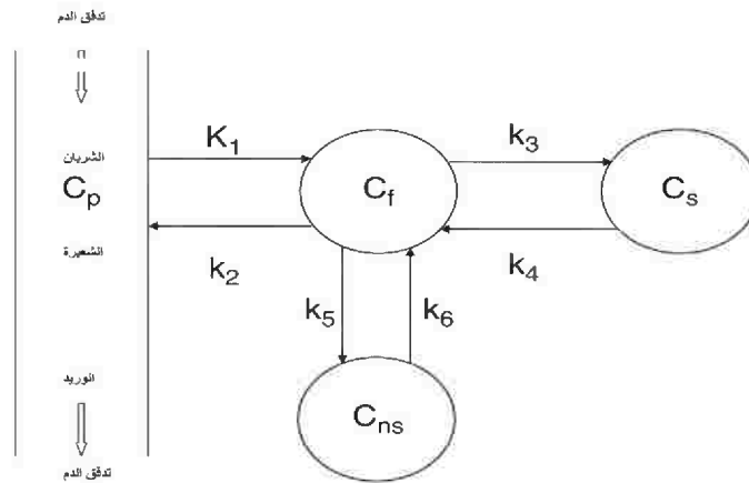
الشكل رقم (٥،١٢) نموذج الحجيرة النسيجي الثالثي.
