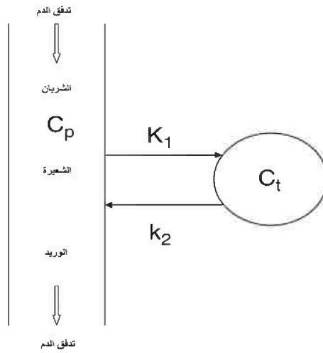
الشكل رقم (٥،٩) نموذج حجرة النسيج الوحيدة.
