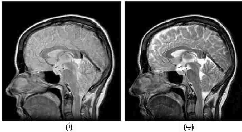
الشكل رقم (١,١٦) صورة شريحة خلال المخ البشري (أ) مع وزن أقل للزمن TE و (ب) وزن زائد للزمن TE.
