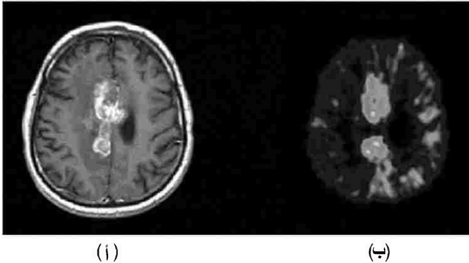
الشكل رقم (٦،١) الفرق بين التصوير الهيكلي (MRI-a) والتصوير الوظيفي (PET-b) في المخ البشري.
