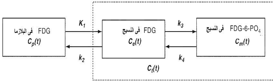
الشكل رقم (٦.٢) نموذج من ثلاث حجيرات وأربعة معاملات لل FDG.
