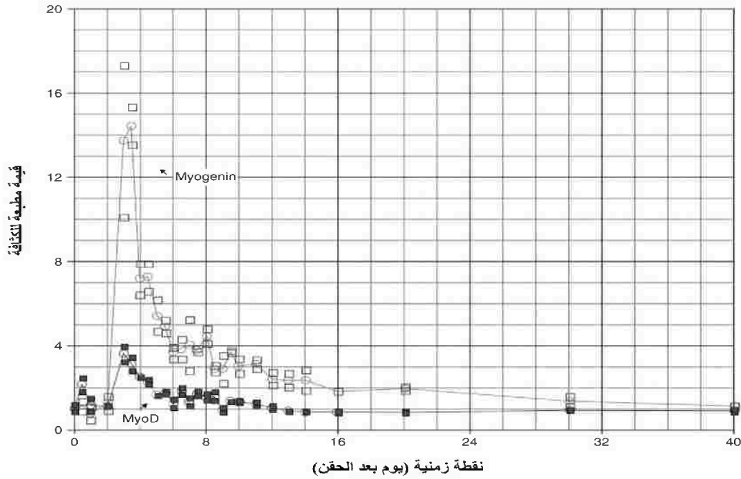
الشكل رقم (١٢،١٣) بيانات المتواليات الزمنية في التجديد العضلي في الجسم الحي (in vivo). هذه البيانات من Zhao et al 2002 [19] and Zhao et al 2003 [18] وهي منشورة في الـ PERP ( http://pepr.cnmcresearch.org ).
