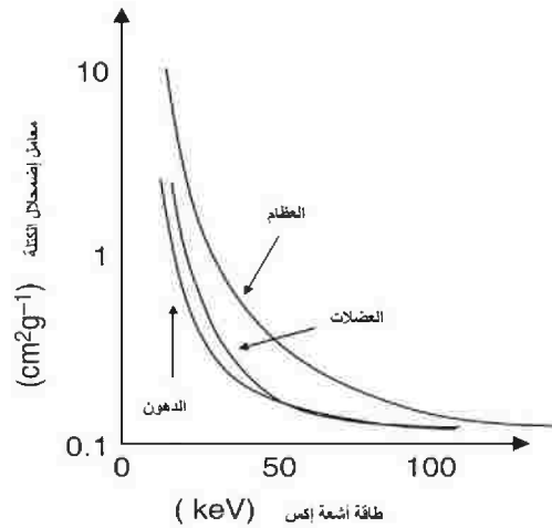
الشكل رقم (١،٢) معاملات اضمحلال الكتلة للعظام والعضلات والدهون كدالة في طاقة أشعة إكس المرسل.
