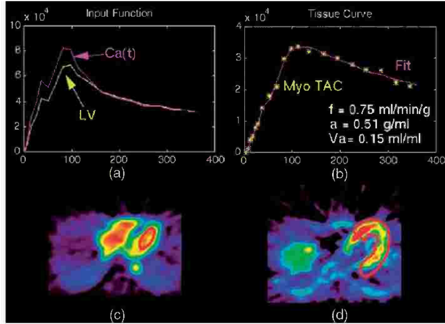
الشكل رقم (٦،١٢) دالة الدخل المستنتجة من صورة للقلب في دراسة ال ^{15}\text{O} -water. الخطوط الحمراء على (c) و (d) تبين حدود منطقة الاهتمام لمناطق الاهتمام ROIs لغرفة البطين الأيسر (c) وللمنطقة المجاورة من عضلة القلب (d). ال LV هو منحنى النشاط الزمني للبطين الأيسر (a) ، وال MyoTAC هو المنحنى لنسيج العضلة القلبية (b) ، و \text{Ca}(t) هي دالة الدخل المتوقعة (a).
