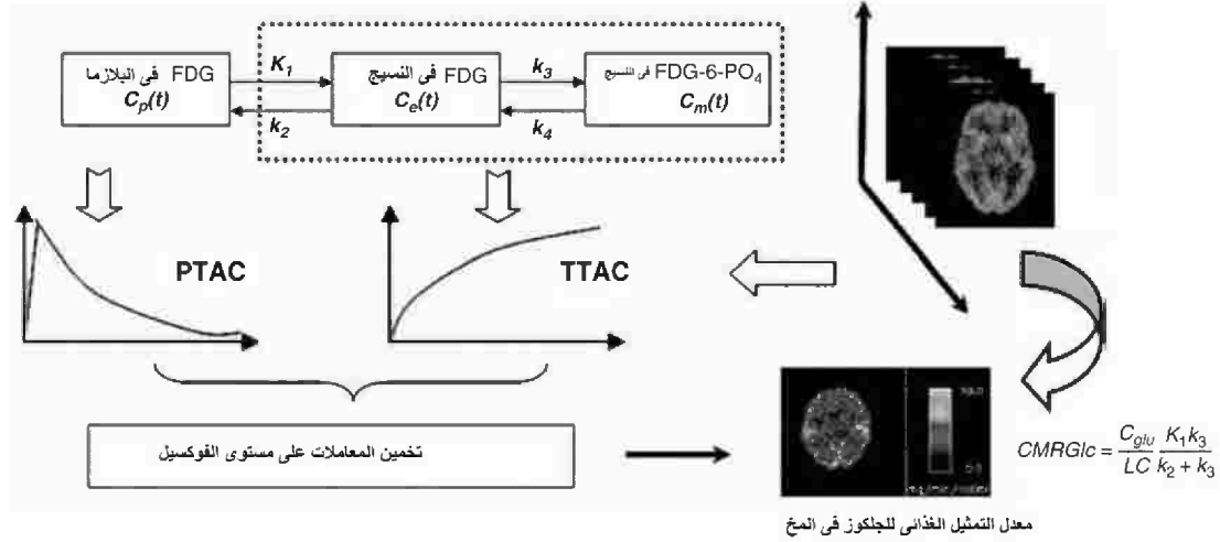
الشكل رقم (٦،٤) مخطط سير لتوليد صورة بارامترية لمعدل التمثيل الغذائي للجلوكوز في المخ CMRGlc.
