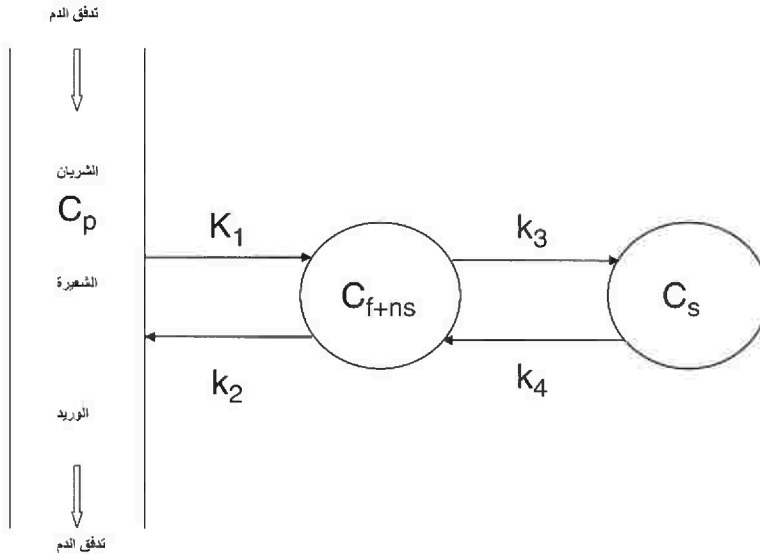
الشكل رقم (٥،١١) نموذج الحجيرة النسيجي الثاني.
