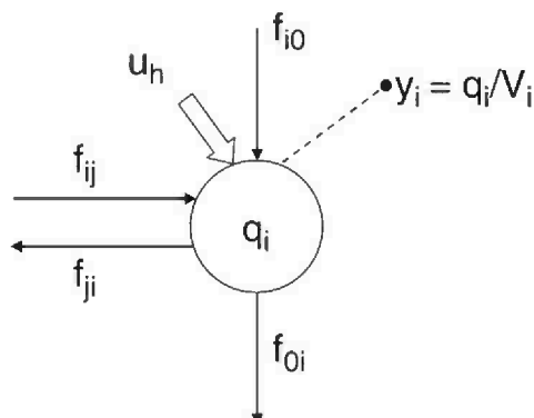
الشكل رقم (٥.٤) الحجرة رقم i في نموذج الأثر المكون من n من الحجيرات مبينا التدفق الداخل والخارج من الحجرة ، والمدخل ، والقياسات.
