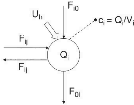
الشكل رقم (٥،٣) الحجيرة رقم i في نموذج من n من الحجيرات يوضح التدفق أو الفيض إلى ومن هذه الحجيرة ، وكل من الدخل والقياسات.
