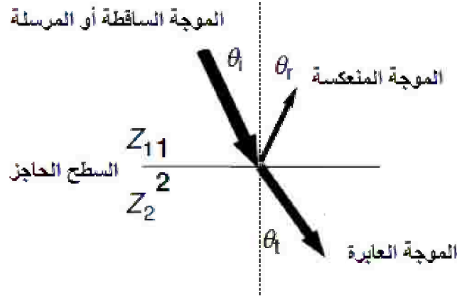
الشكل رقم (١٠، ١) سلوك شعاع فوق صوتي ساقط أو مرسل على السطح الفاصل بين نسيجين بمعاوقة صوتية Z_1 و Z_2 .
