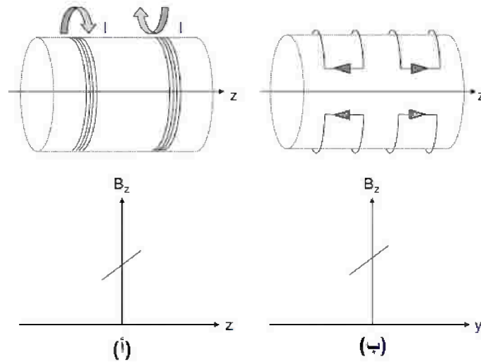
الشكل رقم (١،١٤) (أ) ملفات زوج ماكسويل مستخدمة لإنتاج مجال مغناطيسي خطي في الاتجاه z . (ب) ملفات زوج ماكسويل مستخدمة لإنتاج مجال مغناطيسي خطي في الاتجاه y .
