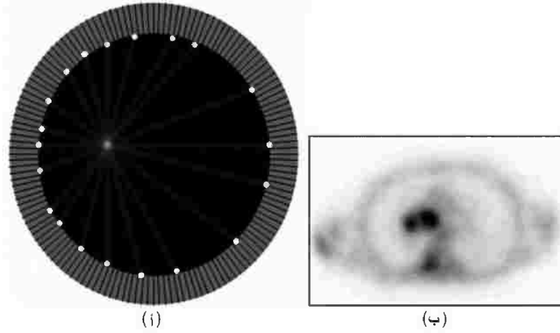
الشكل رقم (١،٨) (أ) تكوين الصورة باستخدام الـ PET. أشعة جاما المتعكسة التوازي تصطدم بزواج من الكشافات التي تكون تكامل خطي للأسقاط العكسي المرشح. (ب) دراسة بطنية بالـ PET باستخدام الـ FDG حيث النقط. الساخنة تبين وجود أورام صغيرة.
