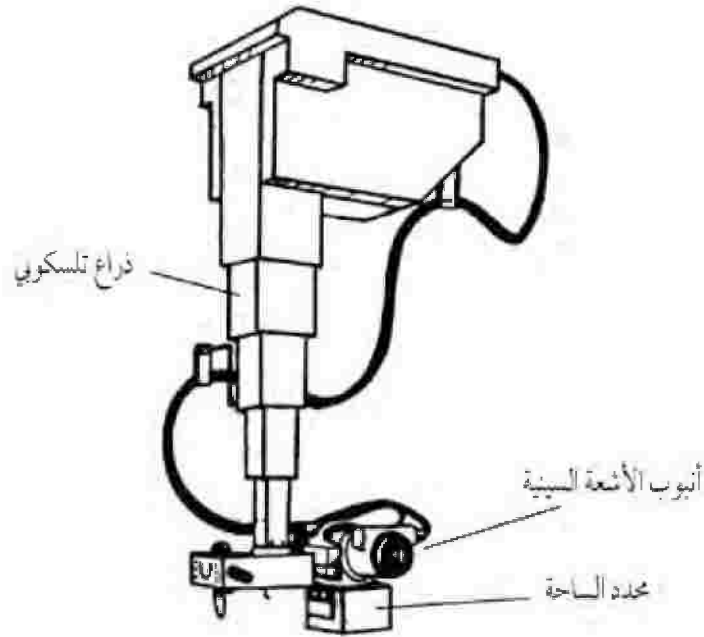
الشكل رقم (١٤). رافعة الأنبوب العلوية. تُستخدم من أجل تموضع أنبوب الأشعة السينية.
