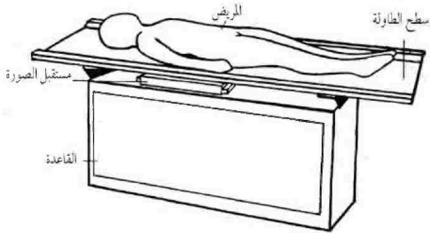
الشكل رقم (١٨). طاولة التصوير الشعاعي. يتحرك مستقبل الصورة و سطح الطاولة لتسهيل التوضع.
