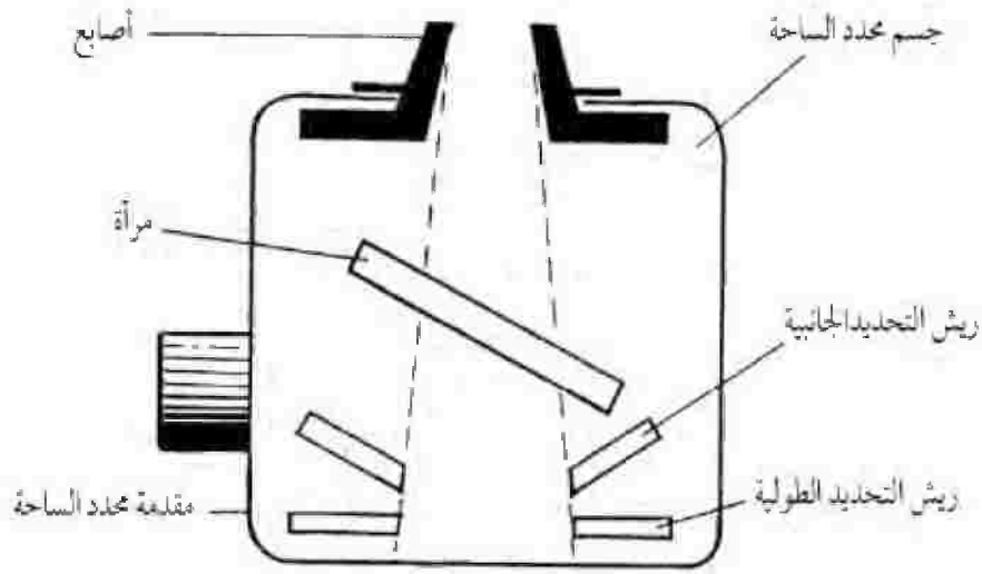
الشكل رقم (١٩). محدد الساحة. إن الأصابع مطلوبة لإزالة الإشعاع الجذعي stem radiation. تضيف المراة ترشيحاً إضافياً لحزمة الأشعة السينية.
