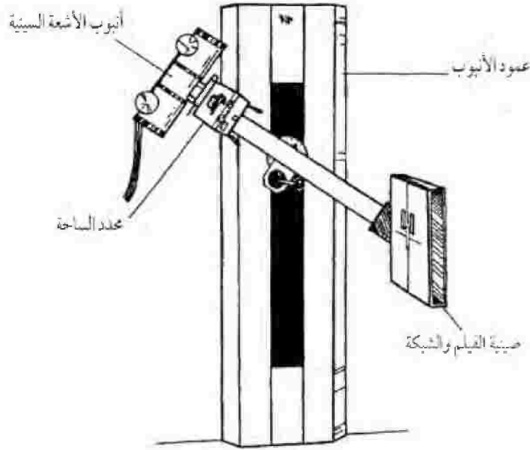
الشكل رقم (١٦). عمود الأنبوب المتكامل. يوضع عمود الأنبوب المتكامل أنبوب الأشعة السينية ومستقبل الصورة أيضاً.
