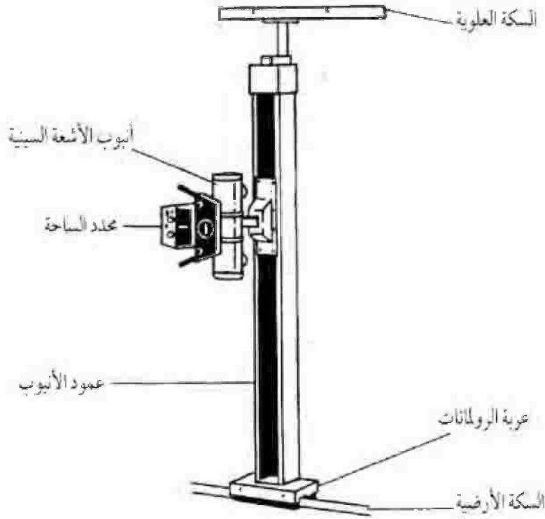
الشكل رقم (١٥). عمود الأنبوب. يُستخدم أيضاً من أجل تموضع أنبوب الأشعة السينية.
