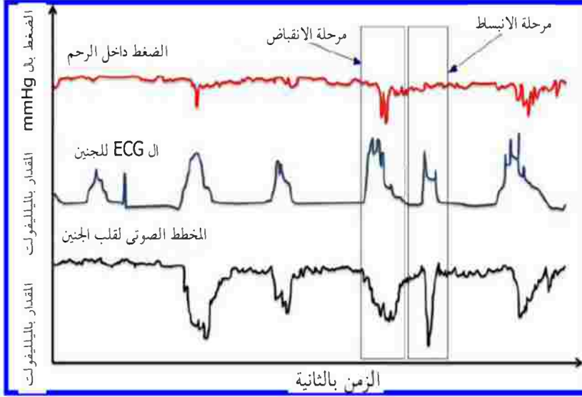
الشكل رقم (٧، ١). يوضح رسم المخطط الصوتي لقلب الجنين (أعلى) مصاحباً لرسم الـ ECG (أسفل) ويمكن ملاحظة الضوضاء في هذا الرسم التخطيطي (المراجع: المراقبة الإكلينيكية للجنين ٢٠٠٤ Fetal clinical monitoring 2004).
