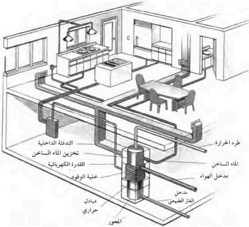
الشكل رقم (٨، ١٢). رسم شطة قدرة مولية [17]. طبع ياذن من إي. سي. لويد.
