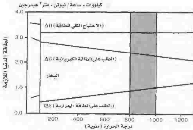
الشكل رقم (٨،٤). الطاقة الدنيا اللازمة لتحليل الكهربائي للماء عند درجات حرارة عالية.
