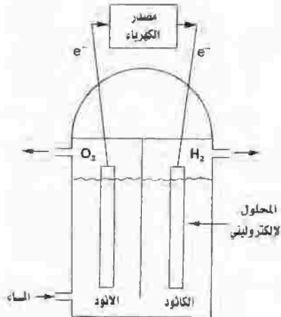
الشكل رقم (٨,٣). رسم توضيحي لخلية تحليل كهربائي قاعدية للماء.
