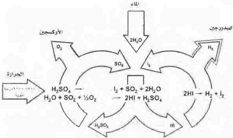
الشكل رقم (٨,٥). رسم توضيحي لدورة الكبريت واليود الكيميائية الحرارية.
