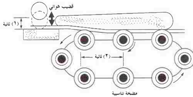
الشكل رقم (١٤,٣). مبدأ التقطيع الهوائي في نظام الجريان المستمر.
