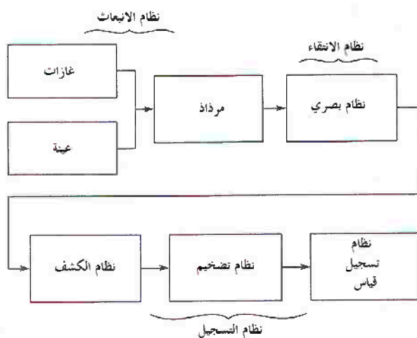
الشكل رقم (١٦، ١٤). الأجزاء الأساسية لقياس ضوء لهي.
