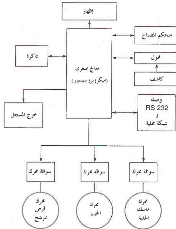
الشكل رقم (١٠، ١٤). مخطط صندوقي لمقياس طيفي ضوئي يتم التحكم به بمعالج صغري.
