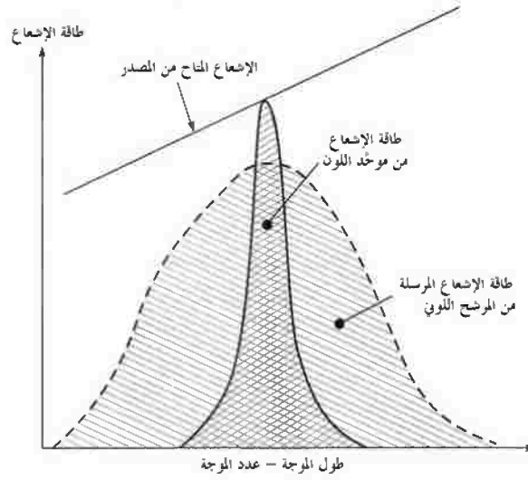
الشكل رقم (٩، ١٤). مقارنة بين طاقة الإشعاع من موحد لون ومن مرشح لون.
