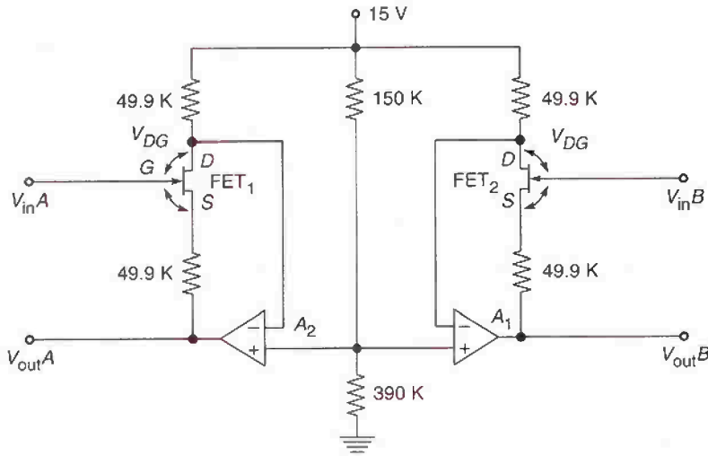
الشكل رقم (١٤,٢٠). مضخم دائري دخل لخلل أيونات.
