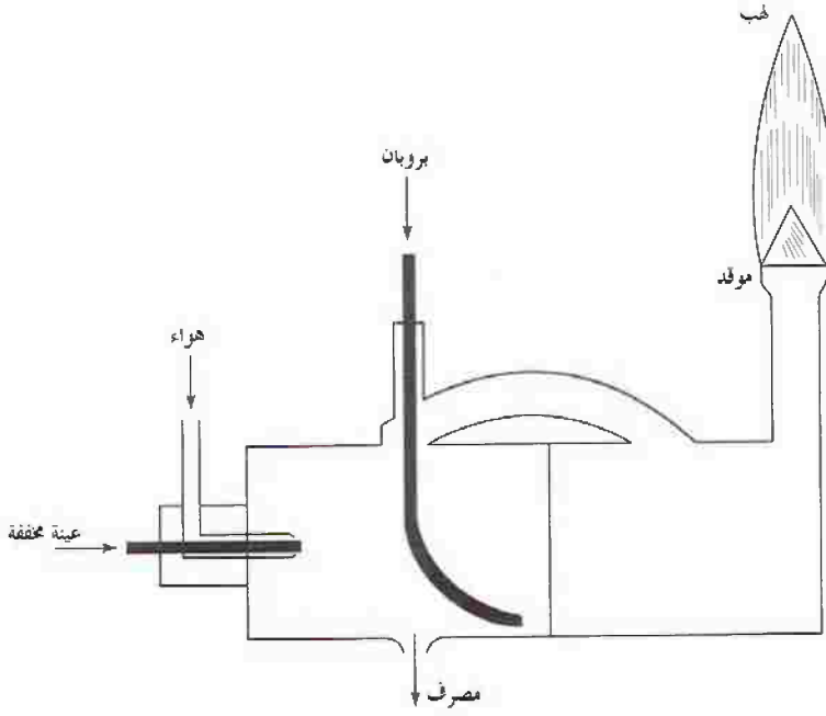
الشكل رقم (١٧, ١٤). حجرة وموقد رذاذ لهب لمقياس ضوء لهبي موديل KLiNa (بموافقة M/s Beckman Instruments)
