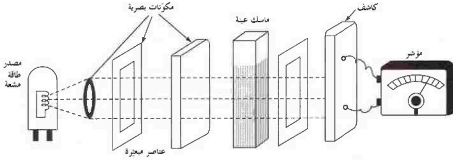
الشكل رقم (١٤, ٢). المكونات المختلفة لجهاز من نوع مقياس طيفي ضوئي.
