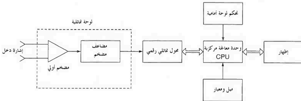
الشكل رقم (١٩، ١٤). مخطط صندوقي لمحلل أيونات بمعالج صغري.
