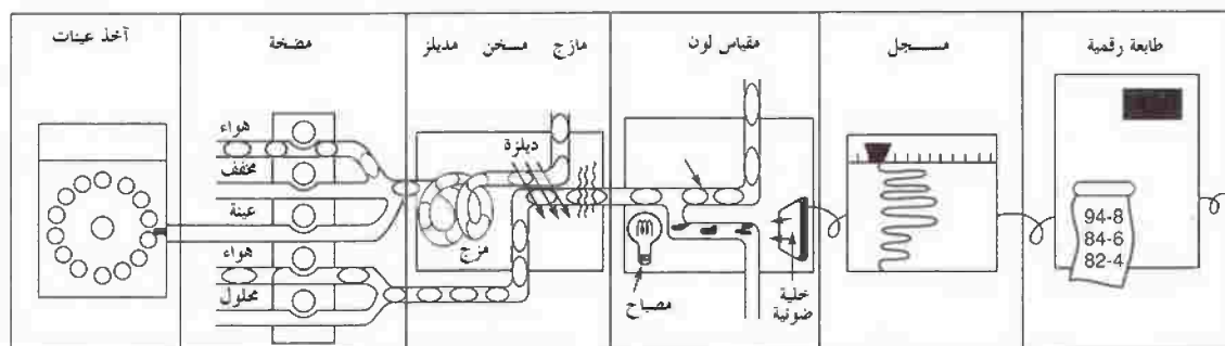
الشكل رقم (١٤, ١١). مخطط تمثيلي لنظام تحليل آلي من النوع ذي الجريان المستمر.
