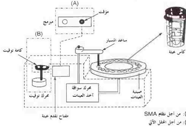
الشكل رقم (١٢، ١٤). متحكمات أخذ العينات (موافقة M/s Technicon Corp).
