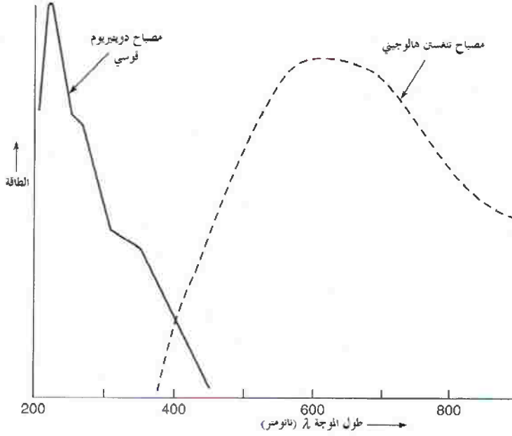
الشكل رقم (١٤,٣). خرج الطاقة كتابع لطول الموجة من أجل مصباح قوس دوتيريوم ومصابيح تنغستن - هالوجين.
