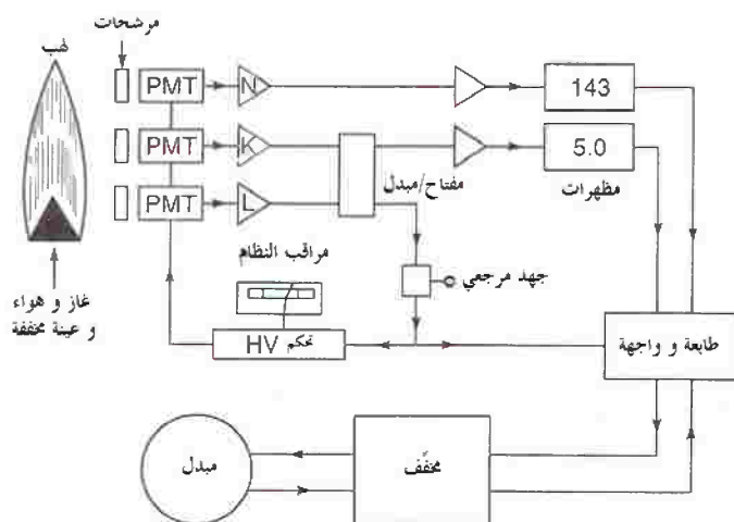
الشكل رقم (١٤، ١٨). مخطط تمثيلي لقياس ضوء لهبي.
