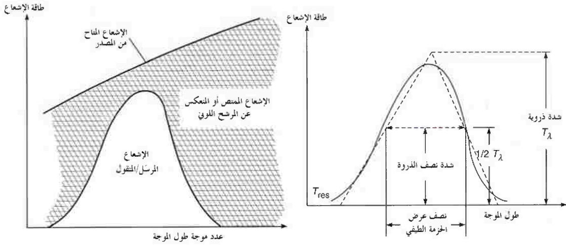
الشكل رقم (١٤،٤). الخواص البصرية لمرشح ضوء.
