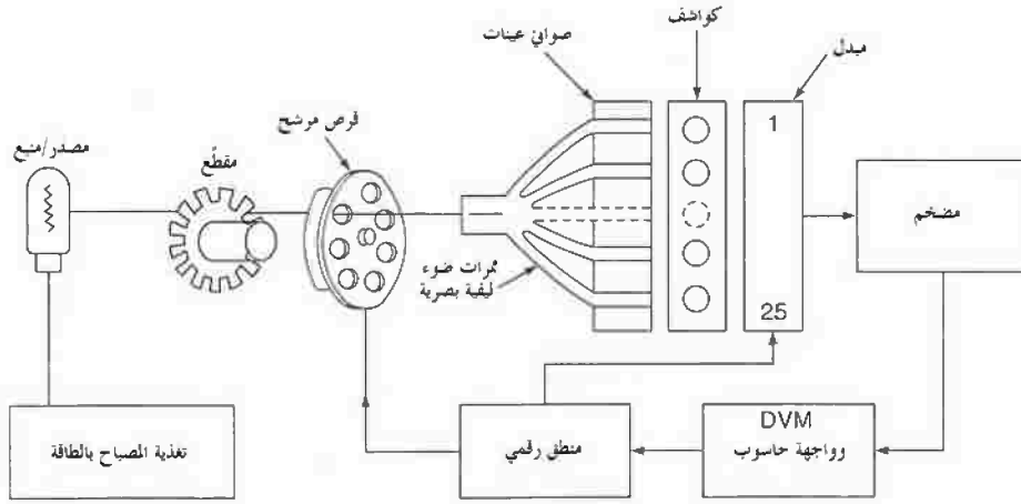
الشكل رقم (١٤,٨). رسم تمثيلي لمقياس ضوء متعدد القنوات.
