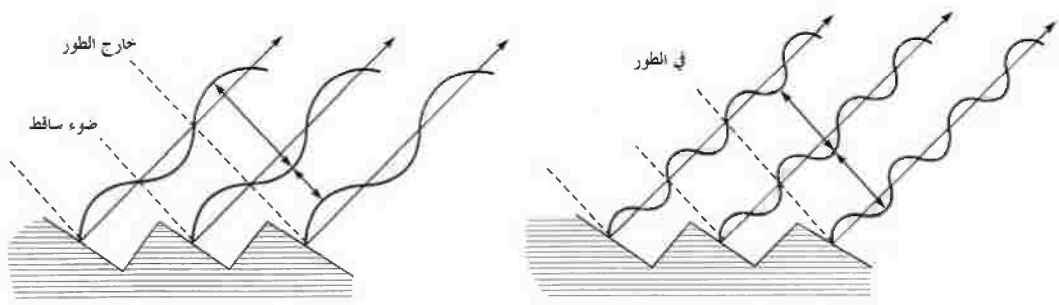
الشكل رقم (١٤, ٦). ظاهرة التبعر في حزيزات الانعراج.
