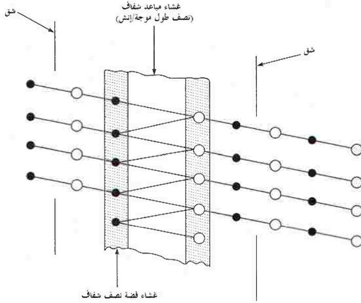
الشكل رقم (١٤,٥). مسار أشعة الضوء عبر مرشح تداخل.
