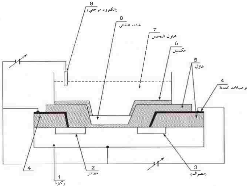
الشكل رقم (١٤،٢١). تفصيلات إنشائية لترانزستور تأثير حقل حساس للأيونات.
