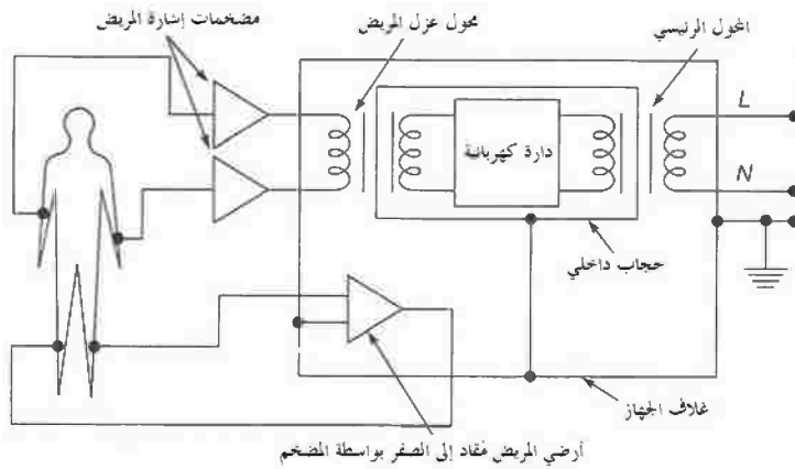
الشكل رقم (٤,٨). مضخم عزل (نوع المحول).
