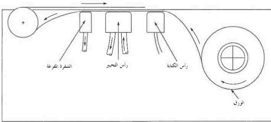
الشكل رقم (٤,٣٠). مبدأ المسجل الكهروستاتيكي. عن (Courtesy: Gould Inc.)
