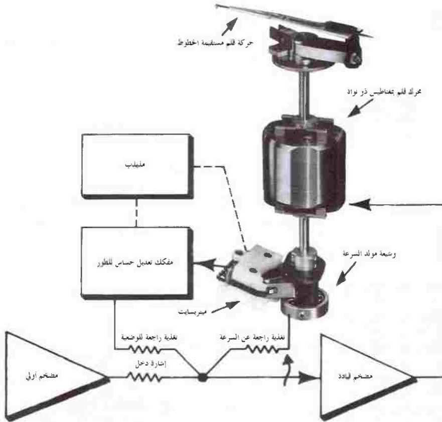
الشكل رقم (٤,٢٥). نظام محرك قلم بتغذية راجعة ذو حلقة سيرفو من أجل تسجيلات سريعة و دقيقة. عن (Courtesy: Gould Inc.)
