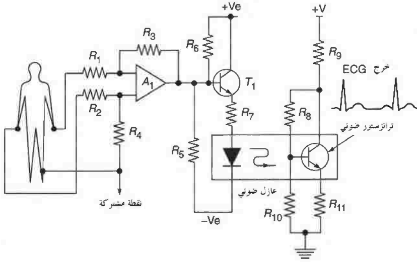
الشكل رقم (٤,٩). مضخم عزل معزول ضوئياً.
