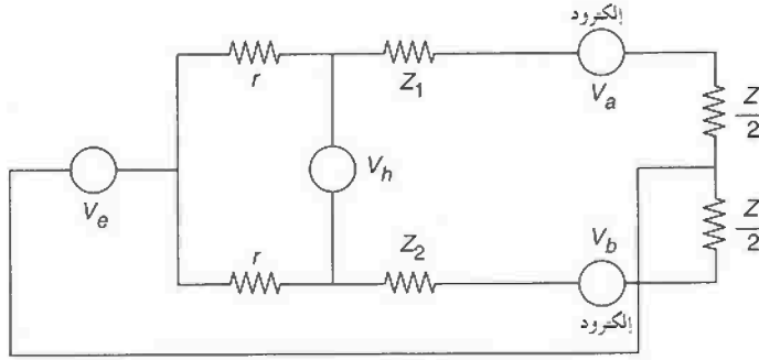
الشكل رقم (٤,٣). دائرة مكافئة للدخل لمضخم ECG.
