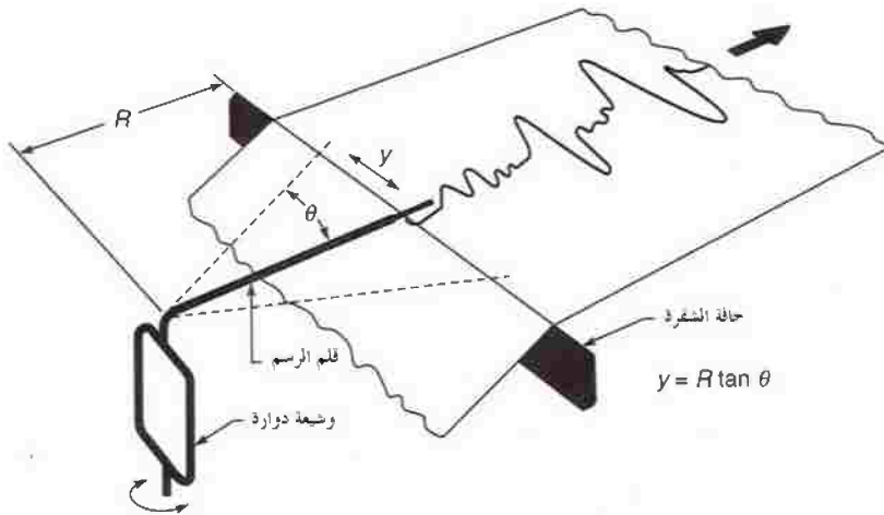
الشكل رقم (٤,٢٣). نظام قلم الرسم المُسخَّن من أجل الكتابة مستقيمة الخطوط على ورق حساس للحرارة فوق حافة شفرة.
