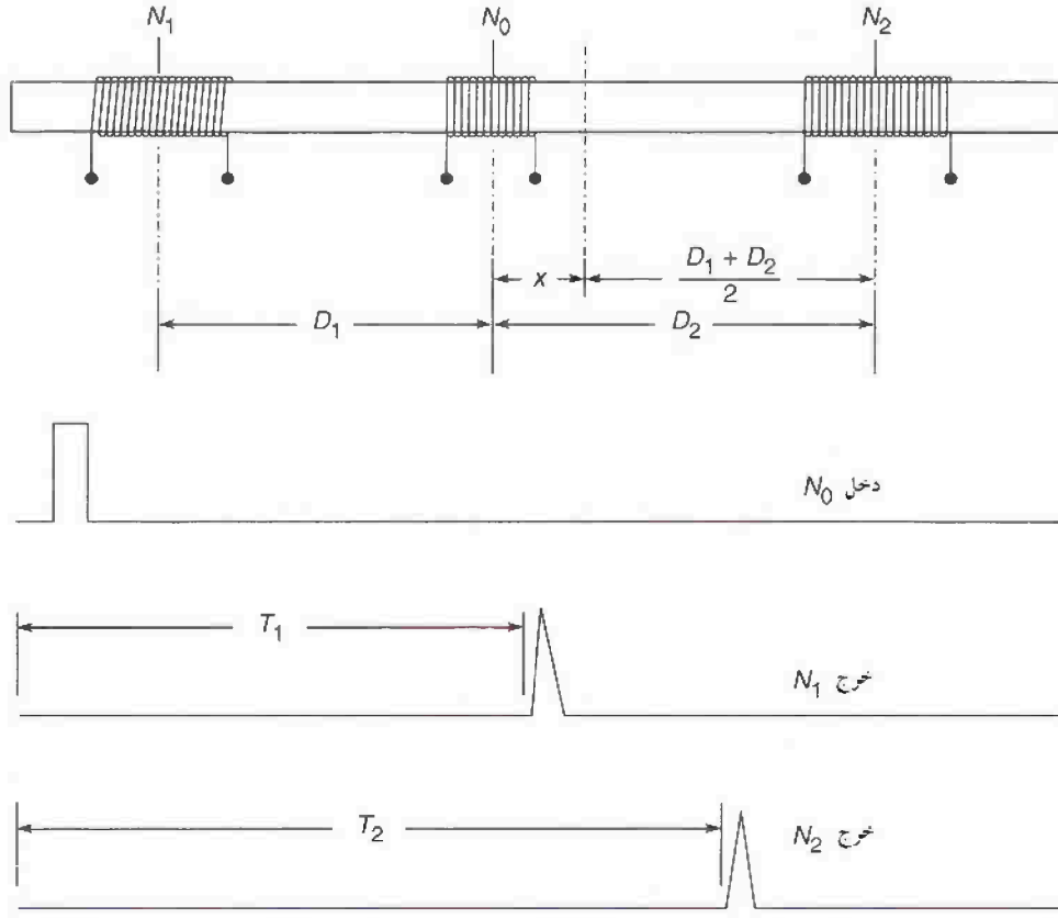
الشكل رقم (٢٨، ٤). مبدل فوق صوتي بتغذية راجعة للوضعية من أجل المسجلات بمقياس الجهد.
