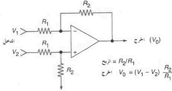
الشكل رقم (٤, ٤). مضخم عملياتي وحيد بترتيب تفاضلي.
