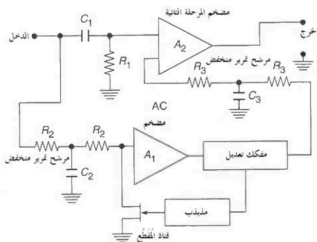
الشكل رقم (٤،٧). مخطط صندوقي مبسط لمضخم عملياتي مستقر مقطع وحيد النهاية.
