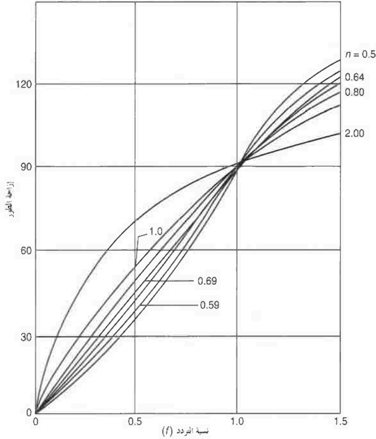
الشكل رقم (٤,٢٠). انزياح الطور بين إشارة القيادة الجيبية وحركة الوشيعة الناتجة كنسبة إلى التردد الطبيعي.
