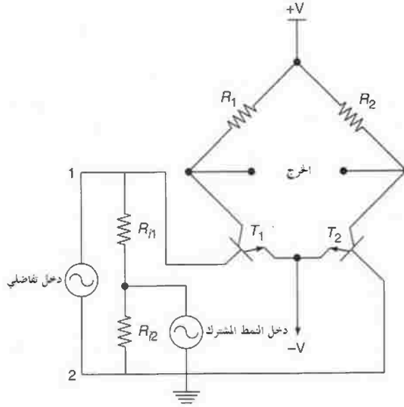
الشكل رقم (٢، ٤). ترتيب لمضخم تفاضلي مثالي.
