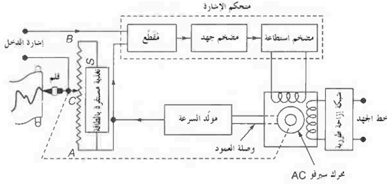
الشكل رقم (٤, ٢٧). رسم تخطيطي لمسجل بمقياس جهد ذاتي التوازن.
