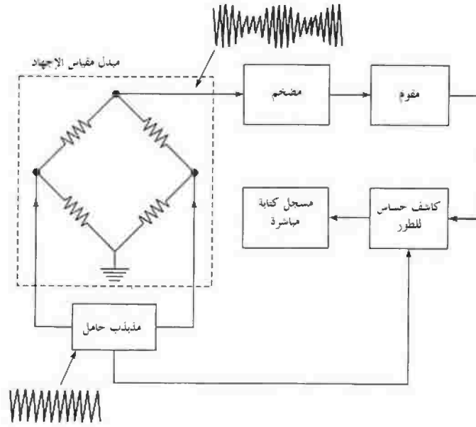
الشكل رقم (٤,٦). مخطط صندوق مضخم حامل.
