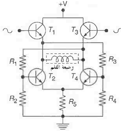
الشكل رقم (٤, ١٧). مرحلة خرج جسرية من أجل وشيعة المقياس الغلفاني القائد في مسجلات الكتابة المباشرة.
