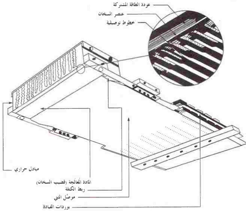
الشكل رقم (٤,٢٩). مبدأ مسجل ذو مصفوفة حرارية. عن (Courtesy: Gould Inc.)
