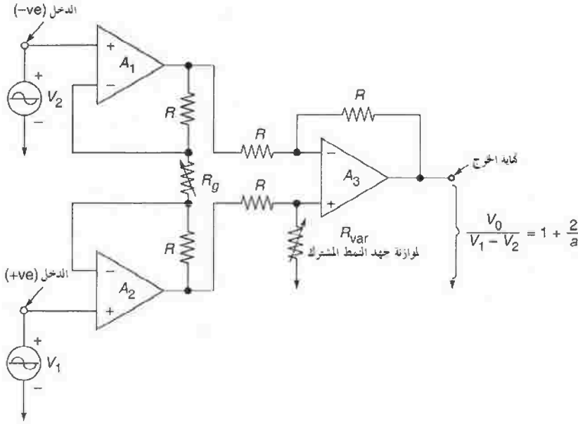
الشكل رقم (٤,٥). رسم تخطيطي لمضخم تجهيزاتي.
