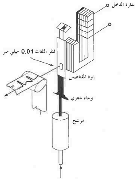
الشكل رقم (٤,٢٦). آلية كتابة بالنفّاث الحبري.
