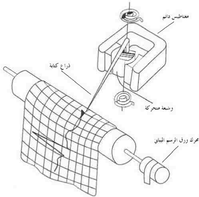
الشكل رقم (١٨، ٤). مبدأ مسجل الكتابة المباشرة بالقياس الغلفاني.
