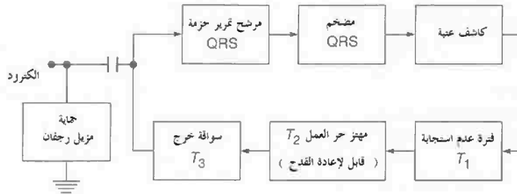
الشكل رقم (٢٥، ٧). مخطط صندوقي لناظم خطى عند الحاجة متزامن بطينياً.
