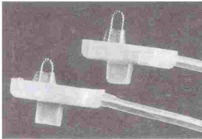
الشكل رقم (٢٥، ١٣). إلكترود عضلة قلبية نموذجي من النوع الحلقي.
