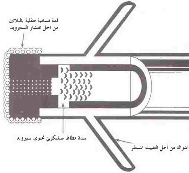
الشكل رقم (٢٥، ١٧). إلكترود ستيرويدي.
