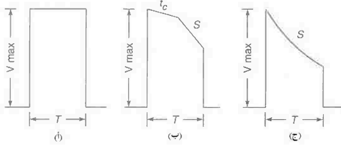
الشكل رقم (٢٥,٣). نبضات من ثلاث أنواع مختلفة من ناظمت الخطى كما تبدو على راسم الإشارة. (أ) ناظم خطى من نوع التيار الثابت. (ب) ناظم خطى فولتي محدود التيار. (ج) ناظم خطى فولتي.
