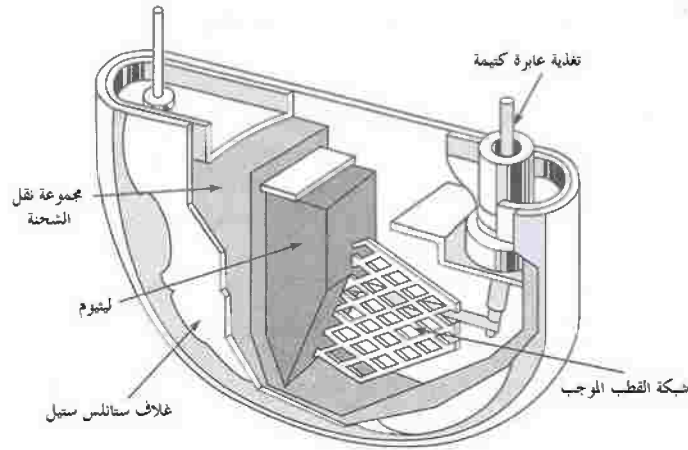
الشكل رقم (٢٥، ١٢). تفاصيل بنيوية لبطارية الليثيوم - اليود. عن (Courtesy: Wilson Greatbatch).
