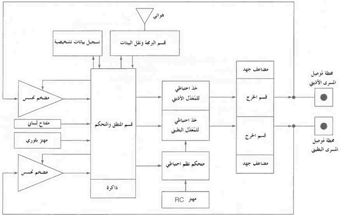
الشكل رقم (٢٥، ١٨). مخطط صندوقي لناظم خطي حديث نموذجي. عن (after Sanders and Lee, 1996).
