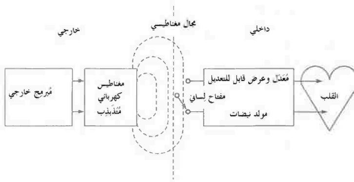
الشكل رقم (٢٥,٨). مخطط صندوقي وظيفي للربط البرمجي.
