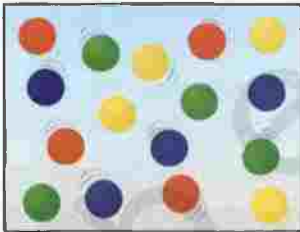
جزيئات سائلة تحركت بعيداً عن بعضها
