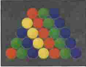
جزيئات صلبة قريبة من بعضها
