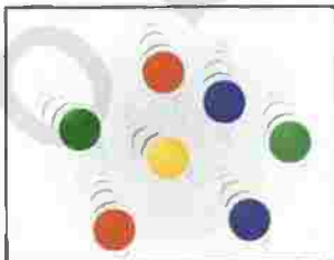
جزيئات غازية تتحرك دائرياً بحرية
