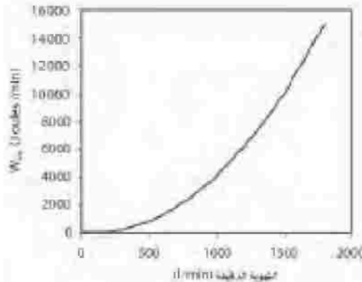
الشكل رقم (٩.٨) العلاقة بين عمل النفس والتهوية مستندة على بيانات من ( Art et al 1990a )
