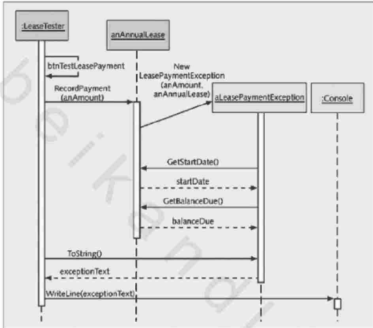
الشكل رقم (٨، ٣٦). نموذج Sequence Diagram يوضح تفاعل إجراء اختبار الصنف LeasePaymentException.
