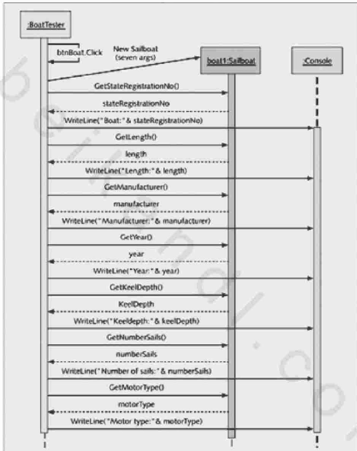
الشكل رقم (١١، ٨). نموذج Sequence Diagram لإجراء اختيار الصنف Sailboat.
