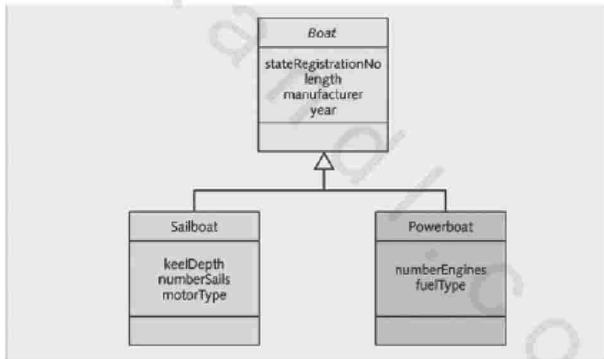
الشكل رقم (٨.٧). شجرة التوارث (التعميم/التخصيص) للصنف المراكب.
