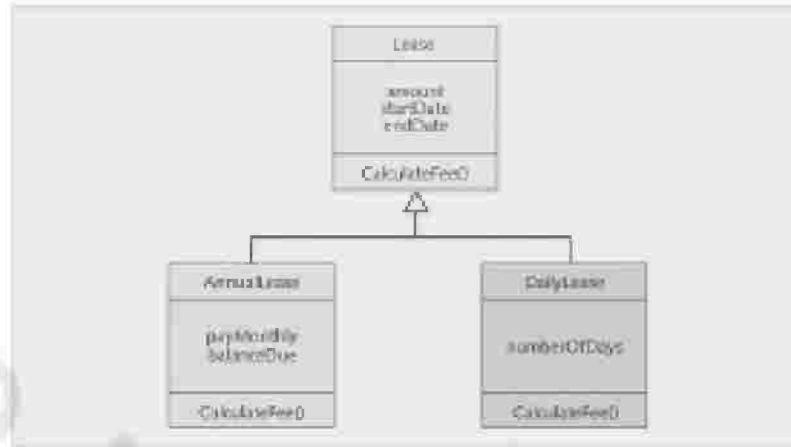
الشكل رقم (٨.١٩). شجرة توارث الصنف Lease.
