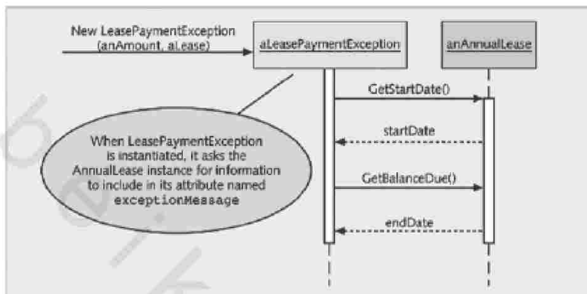
الشكل رقم (٨، ٣٢). نموذج Sequence Diagram يوضح التفاعل بين LeasePaymentException وإجراء الإنشاء.
