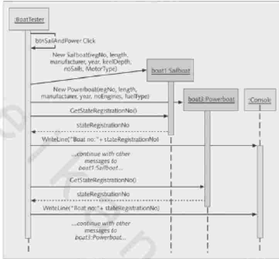
الشكل رقم (٨، ١٥). جزء من نموذج Sequence Diagram لإجراء اختبار الصف Sailboat و Powerboat.
