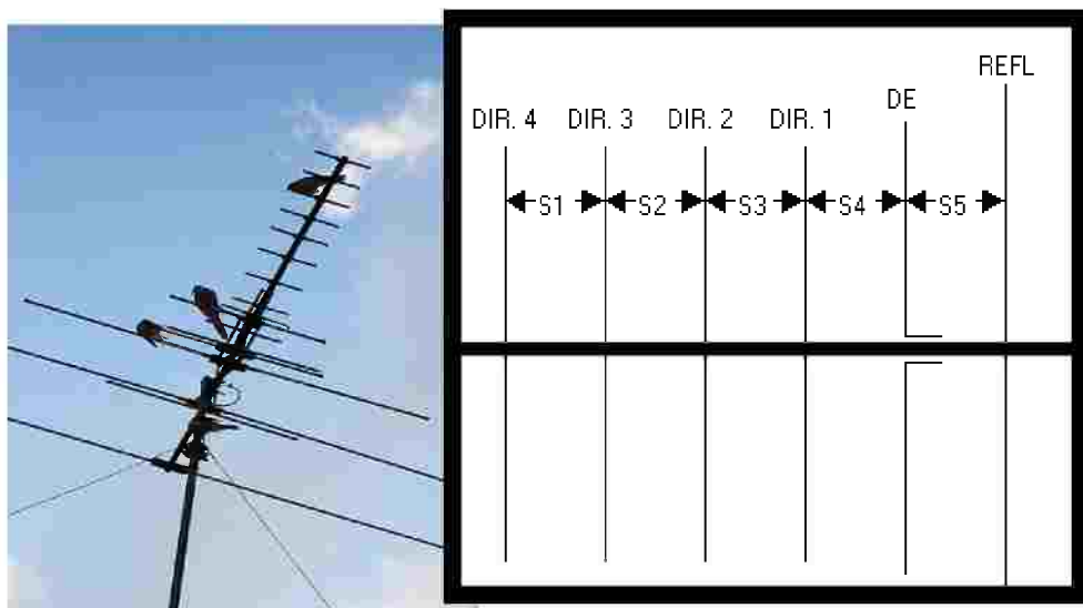
شكل ( 3 - 12 ) هوائي من نوع ياغي
