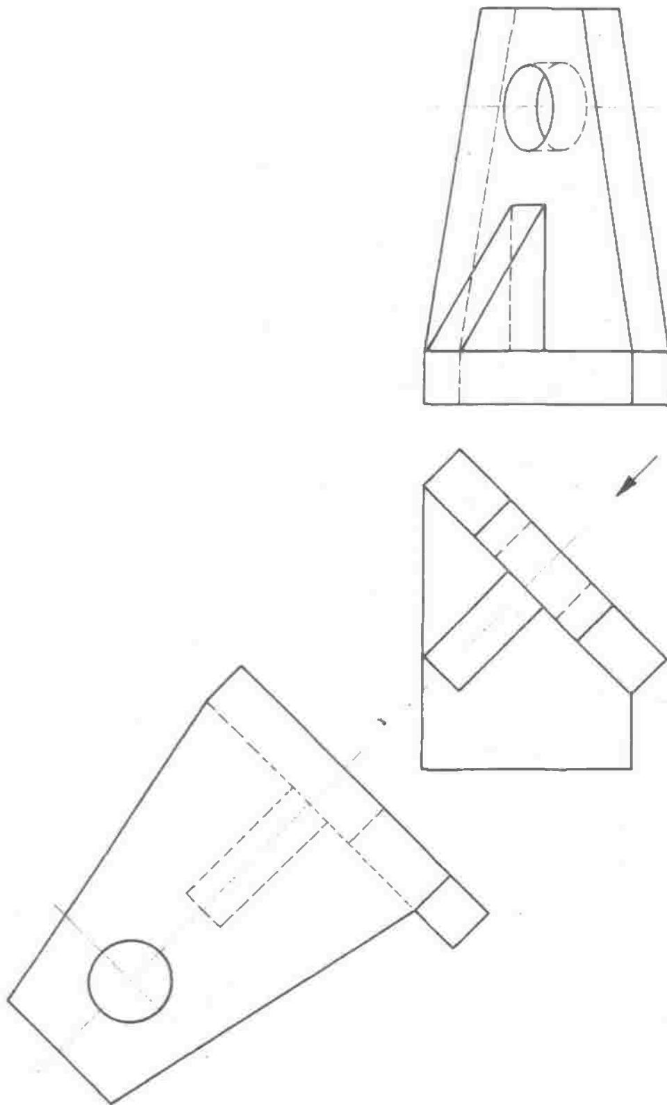
شكل ١٠-٢ « مسقط مساعد للجزء المائل في المسقط الأفقي »
