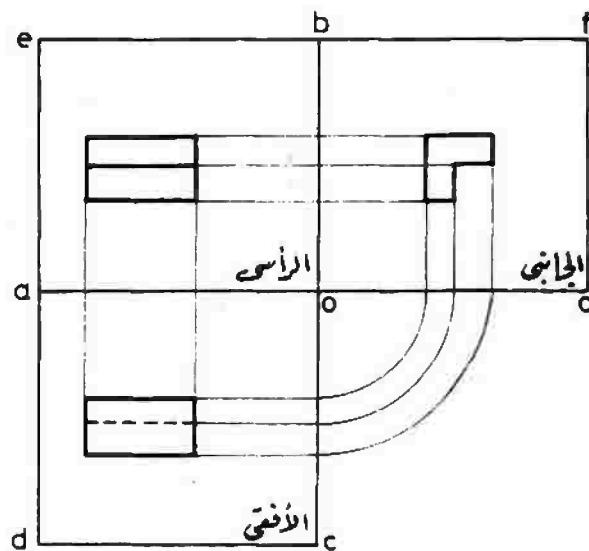
شكل " ٦-٧ " وضع المساقط بالنسبة لبعضها في نظام إسقاط الزاوية الأفقى
