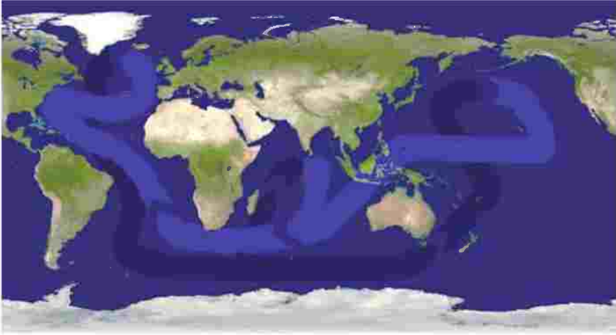
شكل ٢ - ٤ الدورة الحرارية الملحية. تمثل الخطوط الأعمق تيارات المياه العميقة، بينما تمثل الخطوط الأفتح تلك التي تجري على السطح
