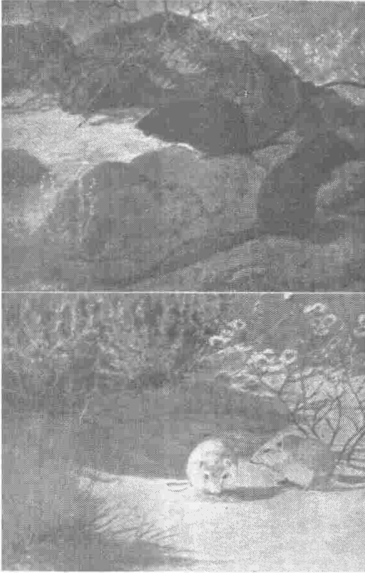
(شكل ٩٠) اكتساب لون البيئة في حيوان « فأر الجيب » في منطقتين متجاورتين ويلاحظ أن النوع المسمى « بيروجناثوس انترميدوس آتر » يعيش فوق صخور الافلا السوداء بينما نوع ب . جيبس يعيش على الرمال الحبيبية البيضاء . (والرسمان من عمل آلات بروك من كتاب بنسون عام ١٩٣٣ بإذن من مطبعة كاليفورنيا)
