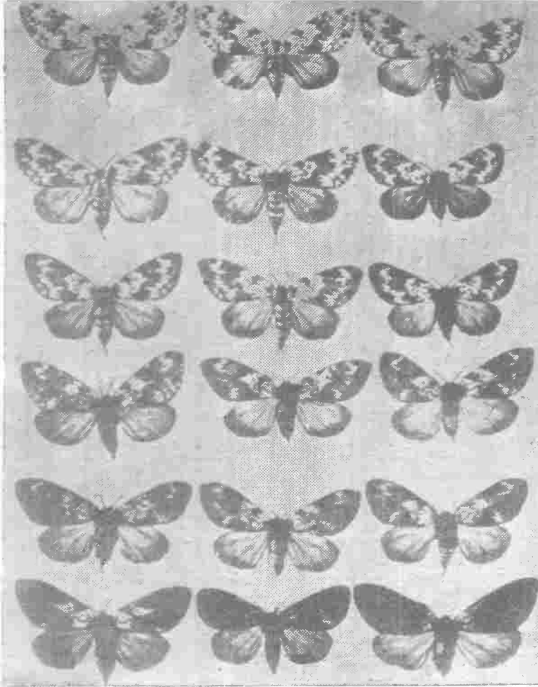
(شكل ٨٩) الميلانية (التلون بالالون الأسود) الصناعية في « ليمانريا موناكا » - يتكون كل صنف من ثلاثة أفراد ويمثل تجمع واحد للزوجين من الجينات الجسدية وزوج واحد من جينات الترابط الجنى الى تسيطر على التلون يمثلون الأسود في هذا النوع .
