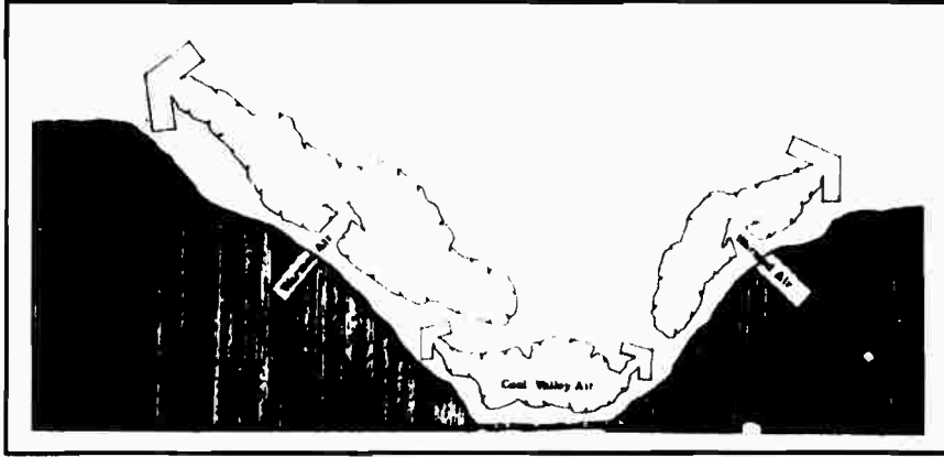
شكل (٨ - أ): نسيم الوادى نهارا، وهو ما يسمى أيضا بالرياح السفحية الصاعدة (١) .
